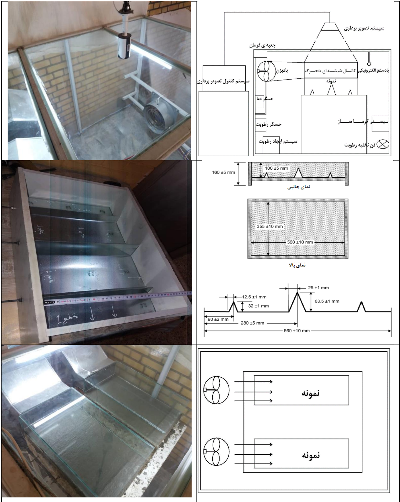
شکل ۴. مشخصات محفظه‌ی شبیه ساز عوامل جوی، قالب و ابزار فولادی استاندارد، نمونه‌های در حال آزمایش
