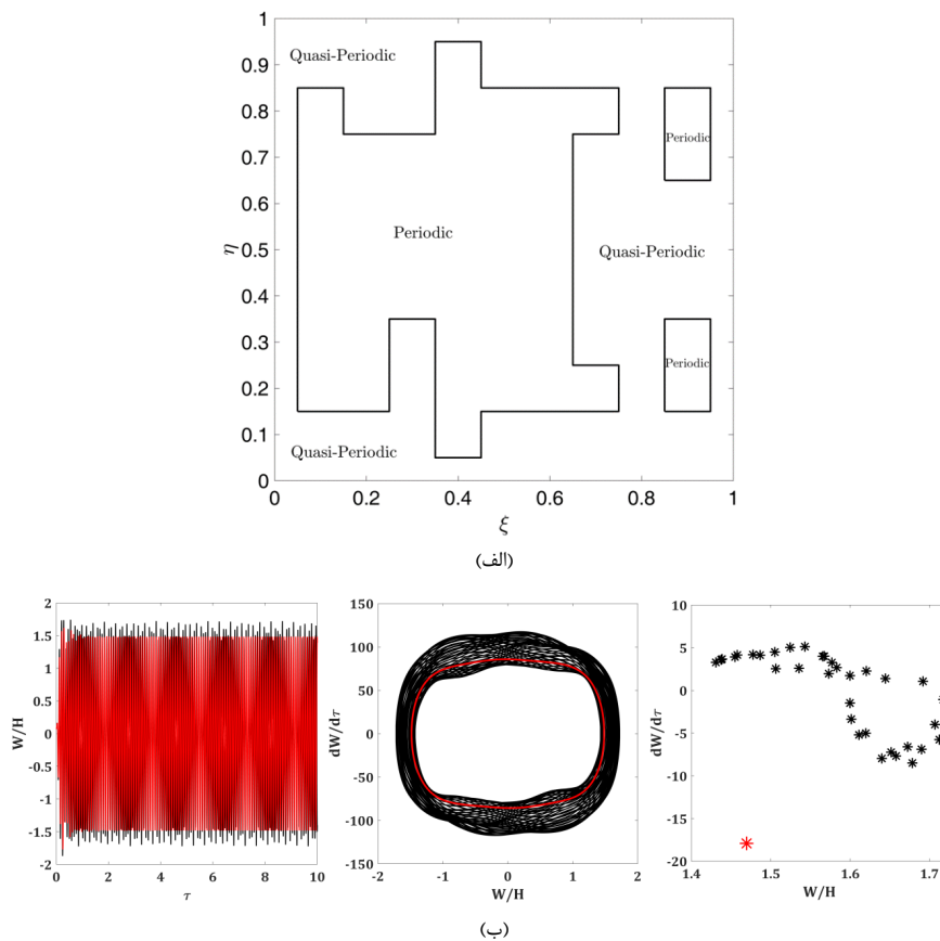
شکل ۶. الف) رفتار ورق الاستیک مربعی با چاه غیرخطی در فشار آبرودینامیک بی‌بعد \lambda = 1280 و \dot{E} = 0 ، ب) نمونه‌ای از تغییر رفتار ورق از شبه‌پریودیک برای ورق بدون چاه به پریودیک برای ورق با نصب چاه در موقعیت [۰.۶، ۰.۴]
