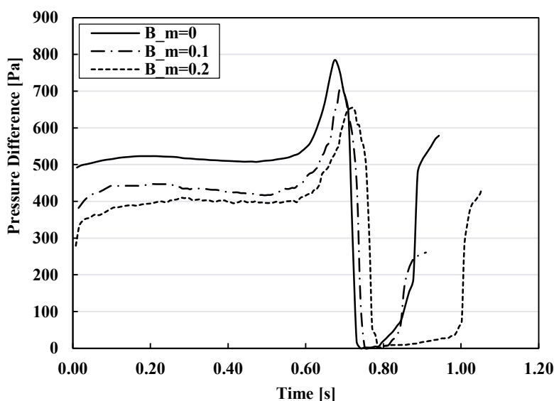
شکل ۹. اختلاف فشار بالادست و پایین دست جریان برای سیال غیرنیوتنی کاریو به عنوان فاز ناپیوسته، تحت شدت میدان‌های مغناطیسی مختلف B_m = 0 و B_m = 0.1 و B_m = 0.2 .
