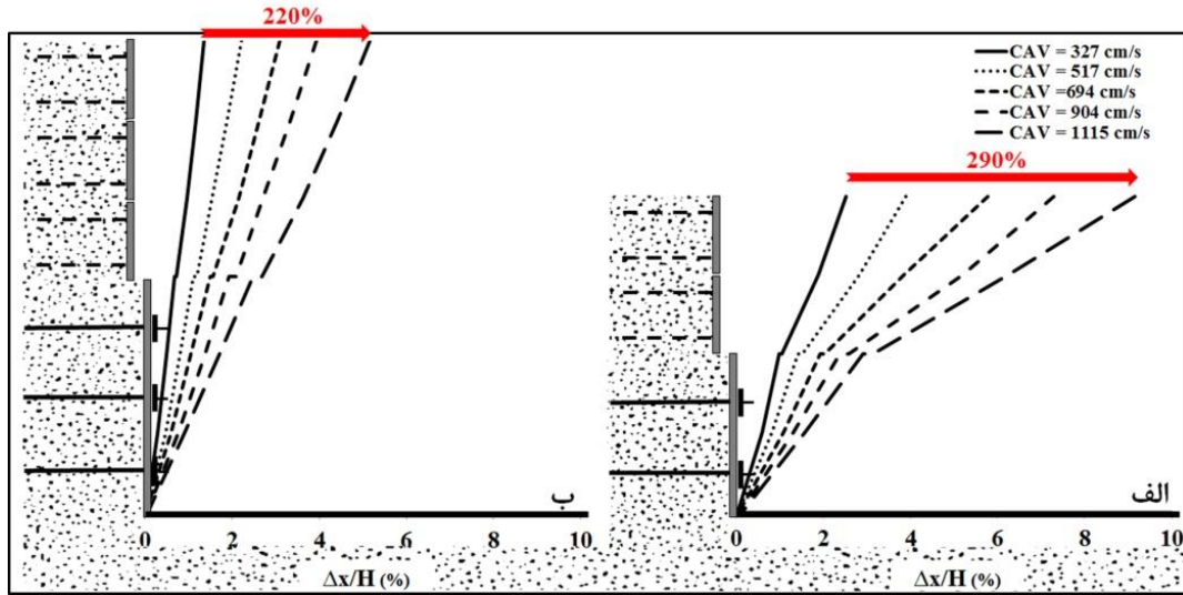
شکل ۲۱. پروفیل تغییر مکان‌های افقی سیستم ترکیبی تحت بار لرزه ای با مقادیر سرعت تجمعی متفاوت: الف) سیستم ۶ متری؛ ب) سیستم ۹ متری
