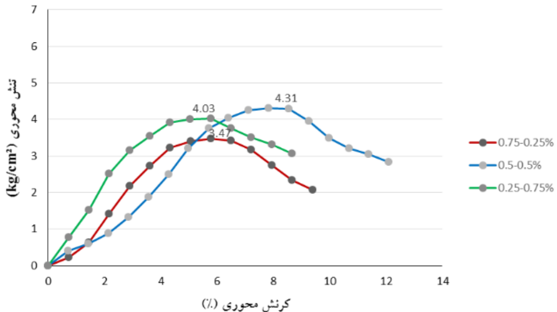
شکل ۱۸. نمودار تنش-کرنش خاک با ترکیب الیاف فولاد صنعتی و پلی پروپیلن
