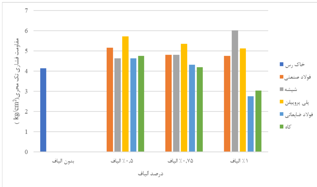
شکل ۱۷. نمودار مقاومت فشاری تک محوری خاک ترکیب شده با پنج نوع الیاف و با درصدهای مختلف به صورت تکی
