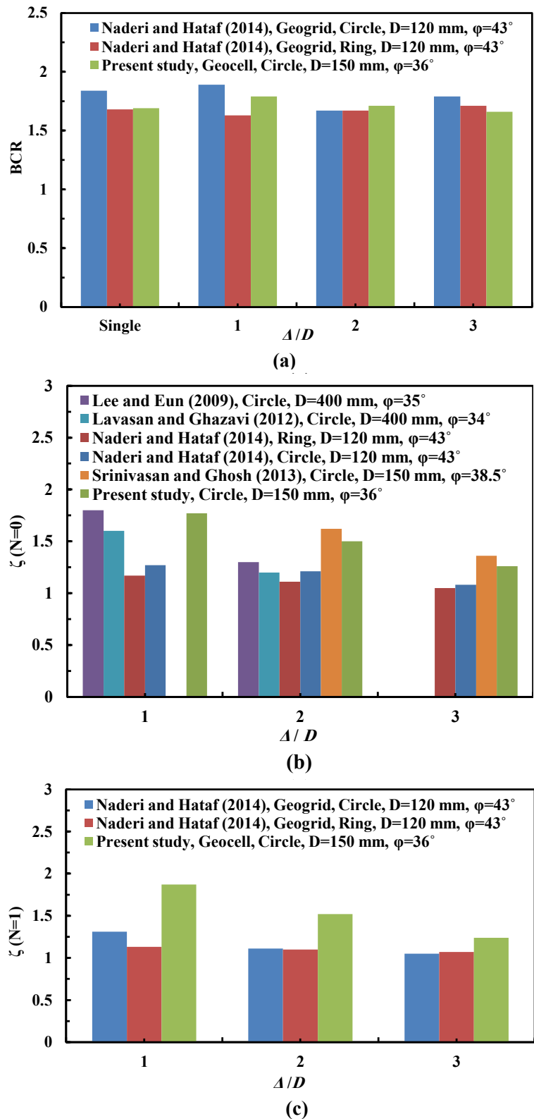
شکل ۸. مقایسه مقادیر BCR و ضریب همجواری ( \zeta ) حاصل از تحقیقات مختلف برای دو شالوده دوار همجواری واقع بر خاک ماسه‌ای: (a) نسبت BCR، (b) \zeta در حالت غیر مسلح، (c) \zeta در حالت مسلح
