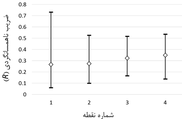
شکل ۷. تغییرات ضریب ناهمسانگردی نرمال برای ۴ نقطه‌ی مشخص شده روی نمودار شکل ۴ Fig. 7. Changes in the normal anisotropy coefficient at the four points marked on Fig. 4
