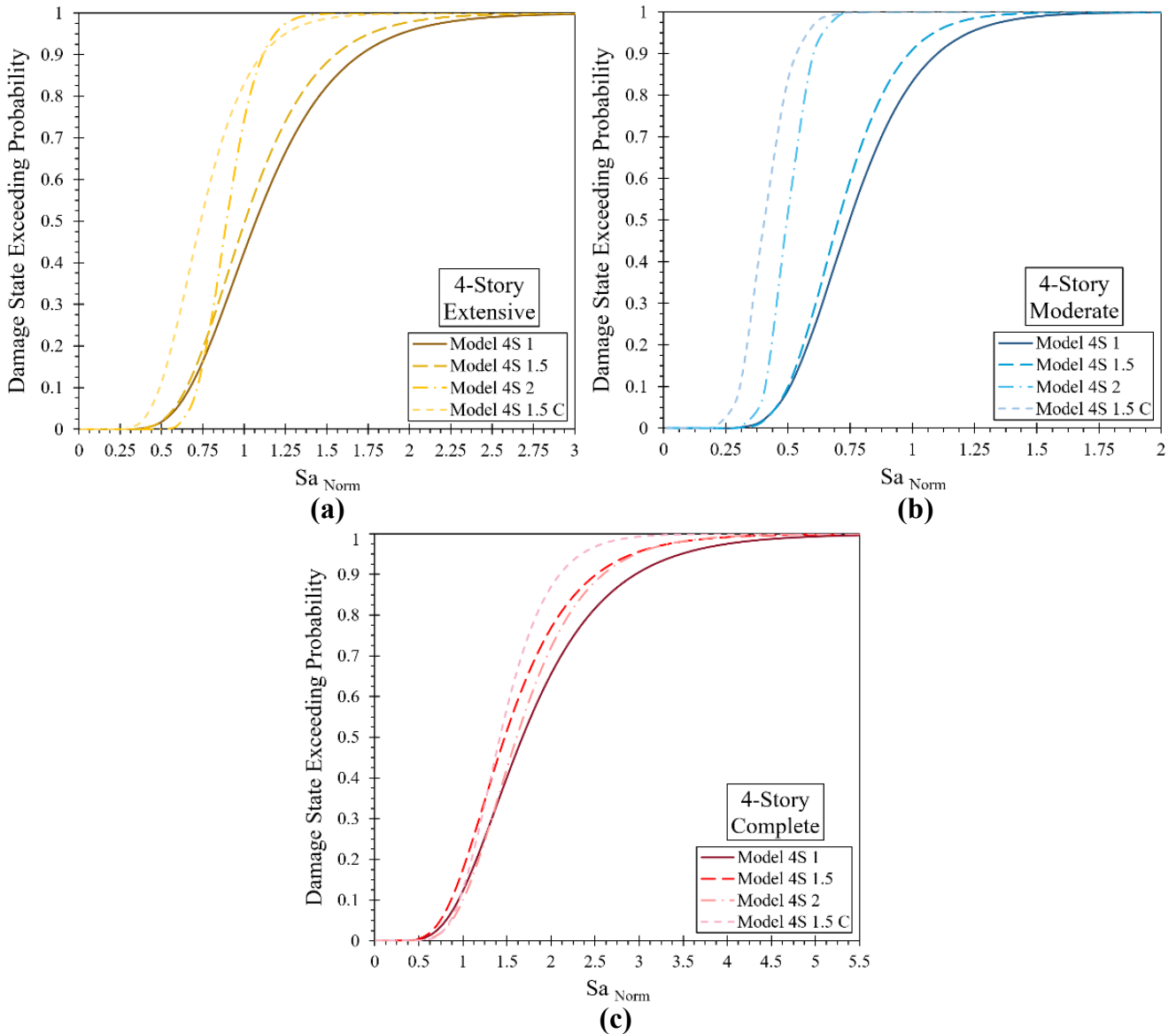
شکل ۱۵. منحنی‌های شکنندگی نرمال شده برای سازه‌های چهار طبقه در سطوح خرابی مختلف (a) متوسط (b) زیاد (c) کامل
