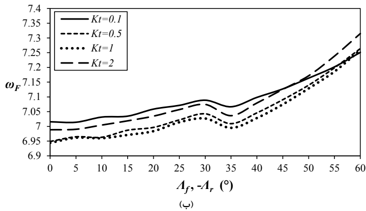
شکل ۹. نمودار اثر زاویه عقبگرد بر (الف) سرعت فلاتر (ب) فرکانس فلاتر بر حسب ضریب سفتی فنر پیچشی
