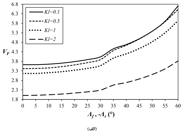
شکل ۱۰. نمودار اثر زاویه عقبگرد بر (الف) سرعت فلاتر (ب) فرکانس فلاتر بر حسب ضریب سفتی فنر طولی
