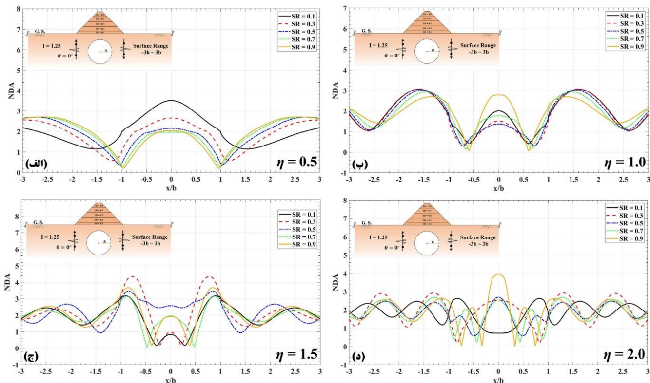
شکل ۳۳. دامنه‌ی تغییر مکان نرّمالایز شده‌ی سطح زمین در مقابل " x/b " برای تپه‌ی آبرفتی دوزنقه‌ای با نسبت امپدانس 1/25 واقع بر حفره‌ی دایره‌ای برای فرکانس بی‌بعد (الف) 0/5 ، (ب) 1 ، (ج) 1/5 و (د) در برابر امواج مهاجم قائم SH.
