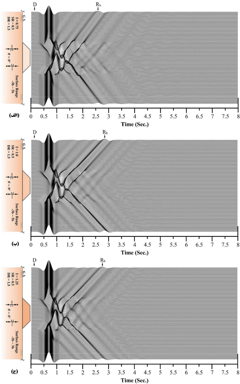
شکل ۸. الگوی کلی پاسخ تاریخچه‌ی زمانی سطح زمین در حضور تپه‌ی آبرفتی دوزنقه‌ای با نسبت شکل ۰/۵ با نسبت امپدانس (الف) ۰/۷۵، (ب) ۱ و (ج) ۱/۲۵ در برابر هجوم امواج قائم SH.
