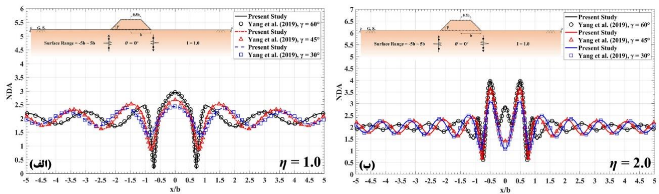
شکل ۴. دامنه‌ی تغییر مکان نورمالایز شده‌ی سطح زمین در مقابل "x/b" برای تپه‌ی آبرفتی ذوزنقه‌ای با زوایای یال (γ) ۳۰، ۴۵ و ۶۰ درجه در فرکانس بی‌بعد (الف) ۱ و (ب) ۲ و هجوم امواج مهاجم قائم SH.
