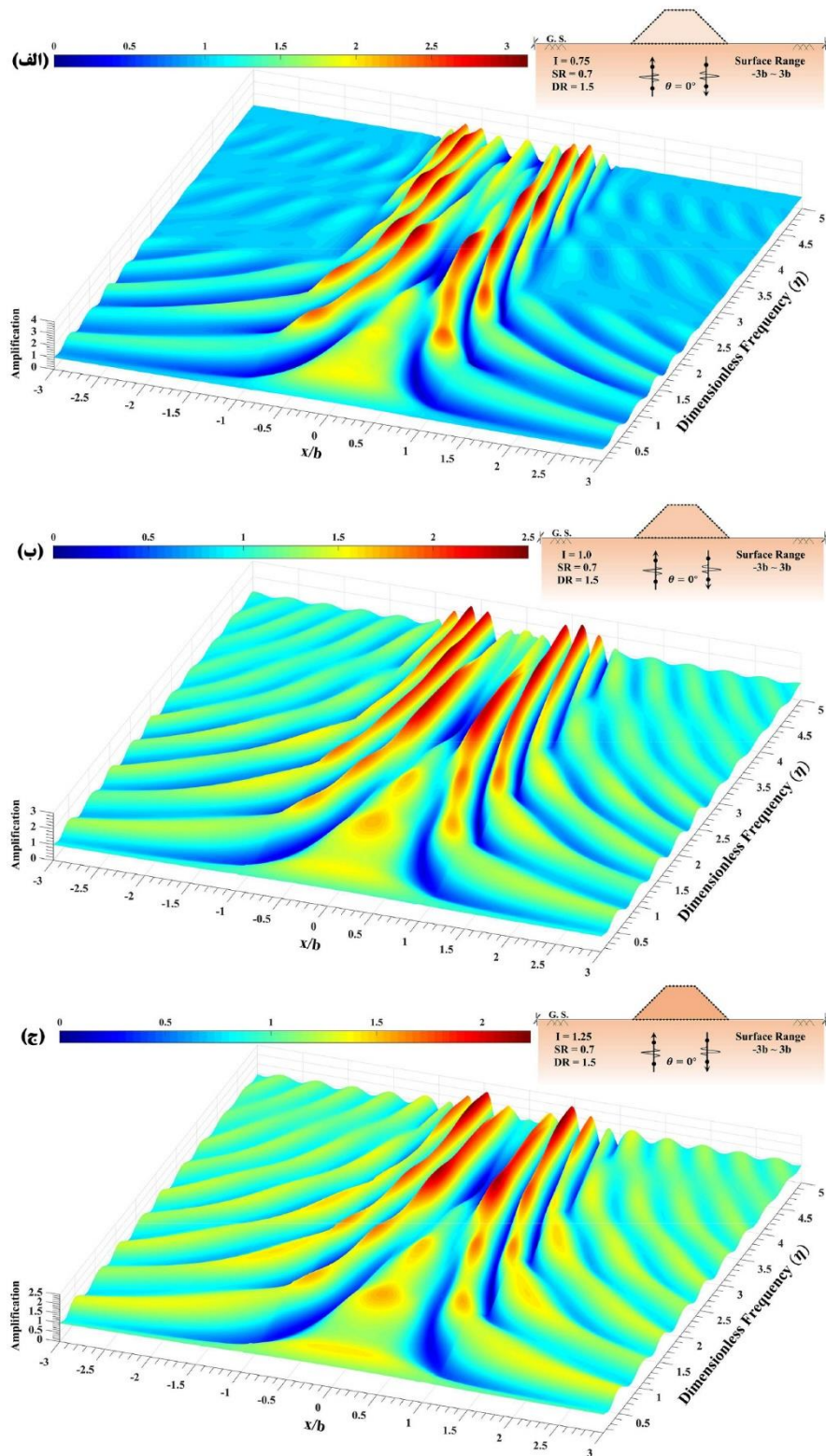
شکل ۲۱. الگوی بزرگ‌نمایی سطح زمین در حضور تپه‌ی آبرفتی ذوزنقه‌ای با نسبت شکل 0.7/1 با نسبت امیدانس (الف) 0.75/1 ، (ب) ۱ و (ج) 1.25/1 در برابر هجوم امواج قائم SH.
