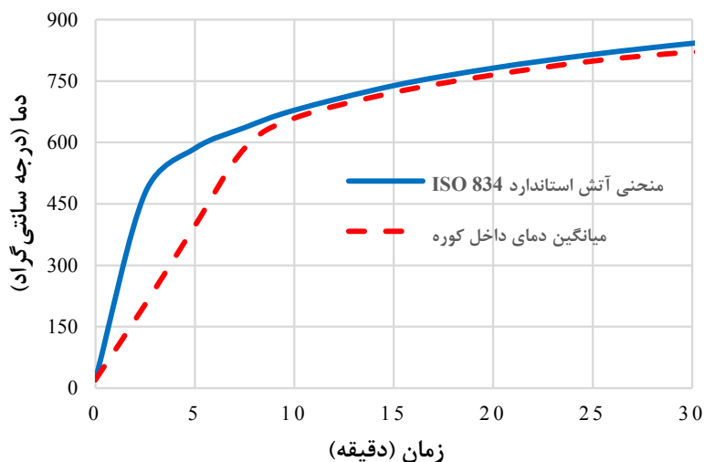
شکل ۴. مقایسه میانگین دمای داخل کوره و منحنی آتش استاندارد ISO 834 [۱۹].
