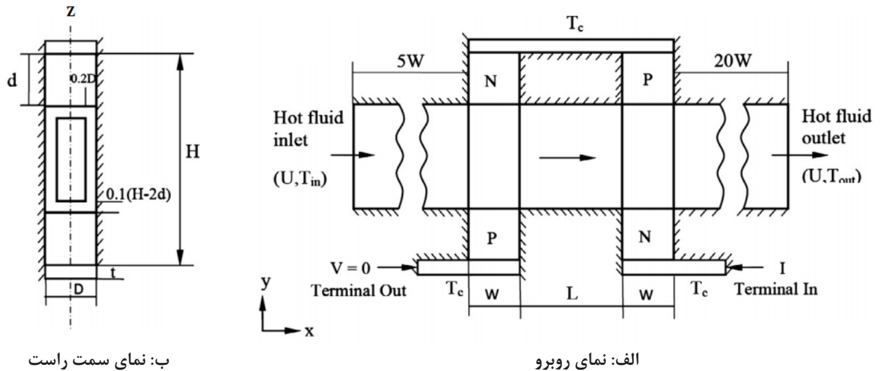
شکل ۱. نمای کلی ترموالکتریک یکپارچه [۹].
