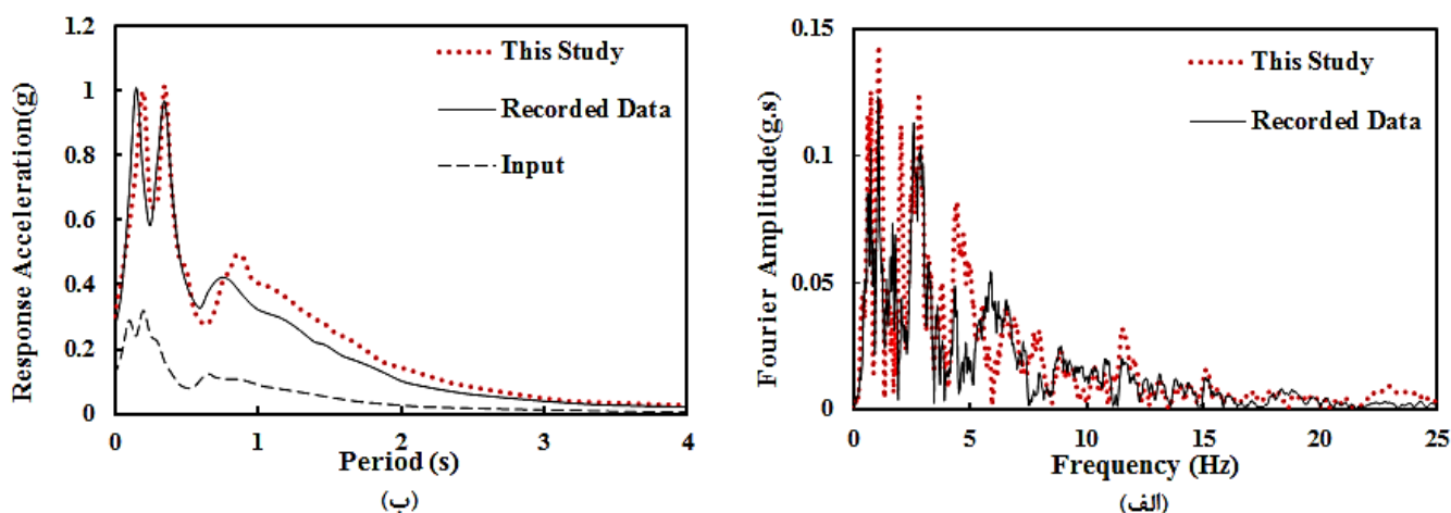
شکل ۸. مقایسه (الف) طیف دامنه فوریه و (ب) طیف پاسخ در سطح زمین، در مطالعه حاضر و نتایج ثبت شده منطقه گیلروی حاصل از زلزله ورودی در سنگ بستر
