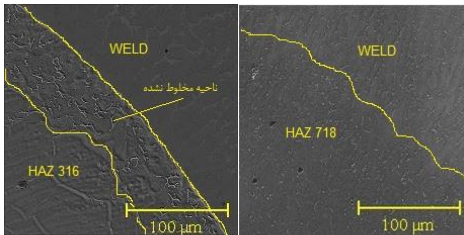
شکل ۱۵. ریزساختار فصل مشترک فلز جوش اینکونل ۷۱۸ با فلزات پایه
