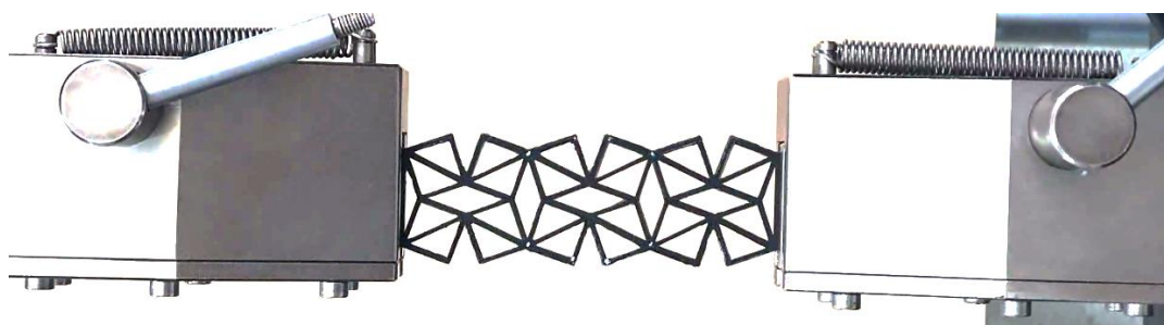
شکل ۵. الف) نمونه چاپ‌شده سه‌بعدی با سه سلول واحد به همراه دو انتها برای نصب در فک‌های دستگاه کشش (ب) نمونه در دستگاه کشش به همراه نقاط کنترل کرنش.
