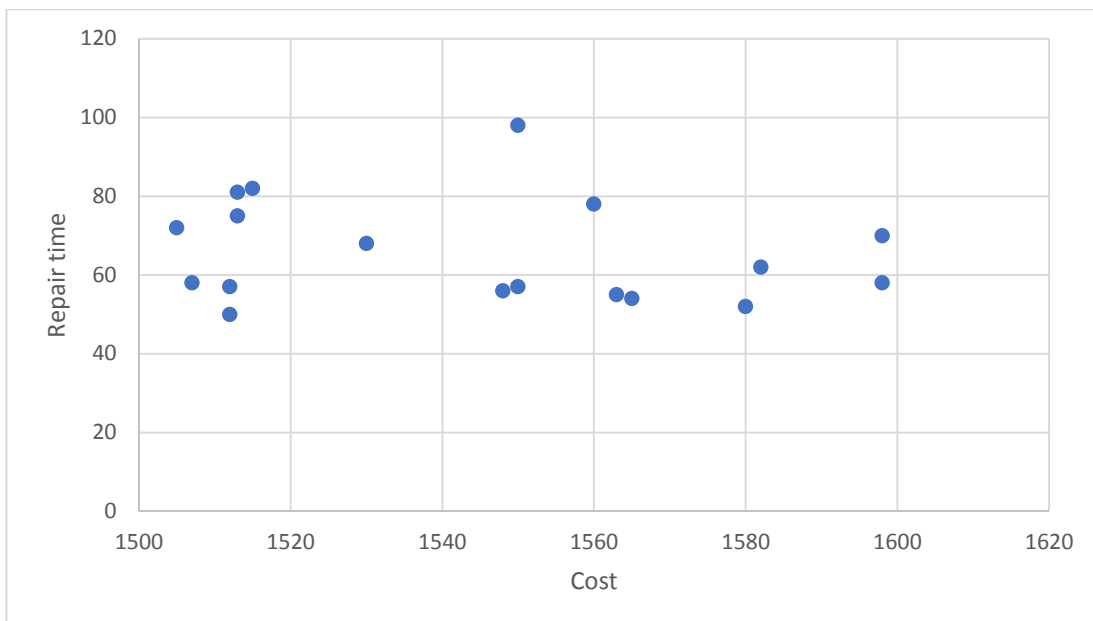
Fig. 7. Pareto frontier
