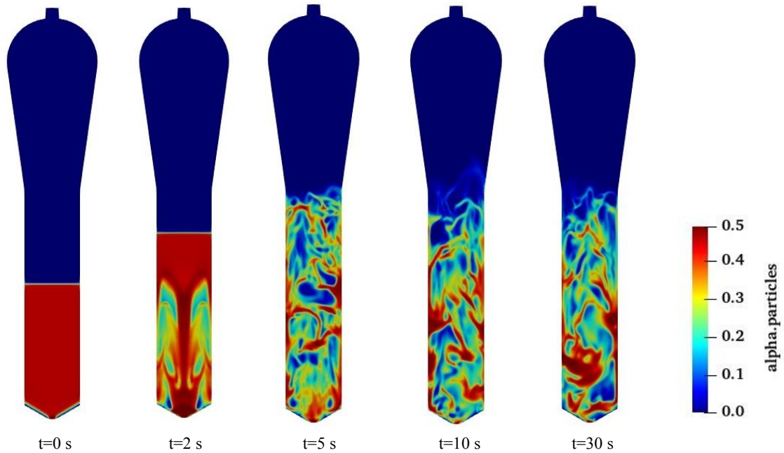
شکل ۸. میدانهای کسر حجمی ذرات جامد حاصل از شبیه سازی راکتور صنعتی مورد استفاده در تکنولوژی بازل در زمانهای مختلف. قطر ذرات جامد: ۱۶۸۵ میکرون، دانسیته ذرات جامد: 918 \text{ kg/m}^3 ، سرعت گاز ورودی: 0.61 \text{ m/s} ، ویسکوزیته گاز ورودی: 1.85 \times 10^{-5} \text{ Pa.s} ، جرم مولکولی گاز ورودی: 40.68 \text{ gr/mol}
