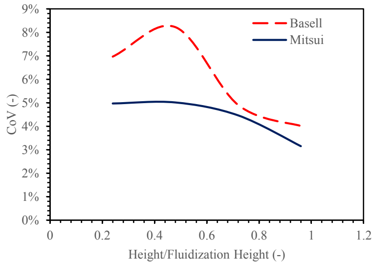
شکل ۱۲. مقایسه ی مقدار ضریب تغییر مربوط به میانگین زمانی کسر حجمی فاز گاز برحسب ارتفاع نرمال راکتور و در دو راکتور مختلف (بازل و میتسوئی). قطر ذرات جامد: ۱۶۸۵ میکرون، دانسیته ذرات جامد: ۹۱۸ kg/m ۳ ، سرعت گاز ورودی: ۰/۶۱ m/s، ویسکوزیته گاز ورودی: ۱۸۵ -۵ Pa.s، جرم مولکولی گاز ورودی: ۴۰/۶۸ gr/mol
