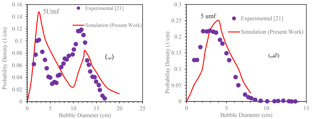
شکل ۶. مقایسه ی توزیع اندازه حبابها در ارتفاع (الف) ۹۰ و (ب) ۲۷۰ میلیمتری از کف بستر و سرعت ۵ برابر حداقل سرعت سیالیت بین داده های شبیه سازی و آزمایشگاهی: ارتفاع راکتور: ۸۰۰ میلیمتر، عرض راکتور: ۱۸۰ میلیمتر، ارتفاع اولیه بستر: ۳۶۰ میلیمتر، قطر ذرات جامد: ۲۵۰ میکرون، دانسیته ذرات جامد: ۲۵۰۰ kg/m ۳ ، حداقل سرعت سیالیت: ۵/۲۴ cm/s، گاز ورودی: هوا. میانگین خطای نسبی شکل الف: ۲۱ درصد و شکل ب: ۴۵ درصد
