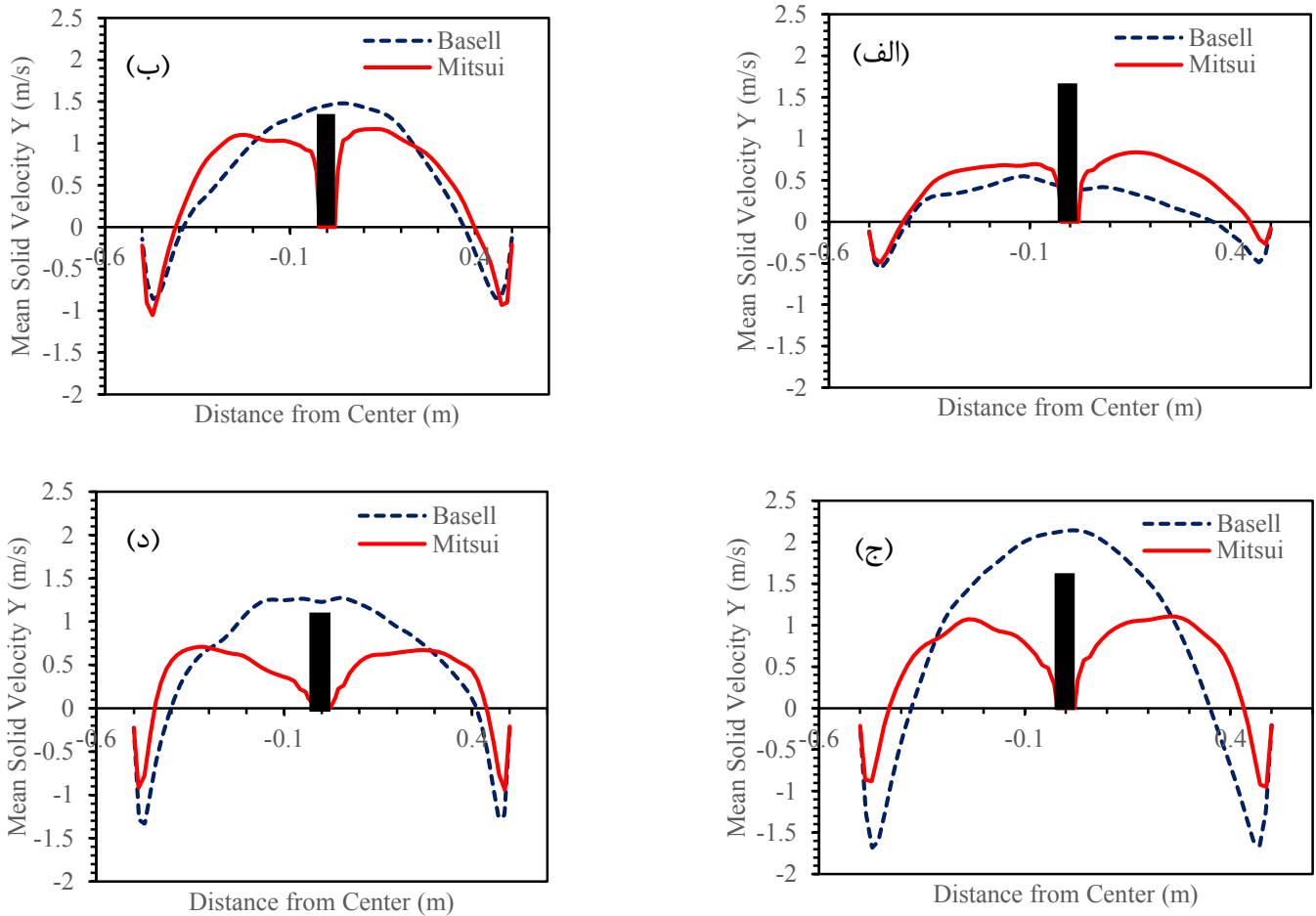
شکل ۱۳. مقایسه‌ی میانگین زمانی سرعت حرکت ذرات جامد (از زمان ۱۰ تا ۳۰ ثانیه) در جهت محوری در دو راکتور مختلف (بازل و میتسویی) و در ارتفاع‌های نرمال مختلف ((الف) ۰/۲۴، (ب) ۰/۴۸، (ج) ۰/۷۲، (د) ۰/۹۶) قطر ذرات جامد: ۱۶۸۵ میکرون، دانسیته ذرات جامد: 918 \text{ kg/m}^3 ، سرعت گاز ورودی: 0.61 \text{ m/s} ، ویسکوزیته گاز ورودی: 1.85 \times 10^{-5} \text{ Pa.s} ، جرم مولکولی گاز ورودی: 40.68 \text{ gr/mol}
