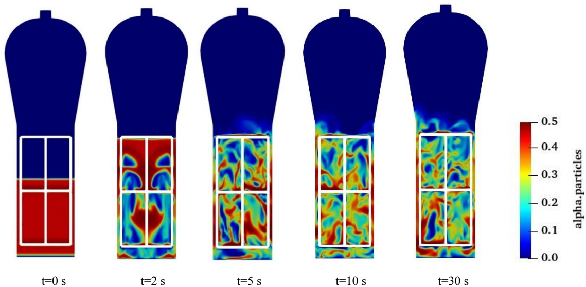
شکل ۹. میدانهای کسر حجمی ذرات جامد حاصل از شبیه سازی راکتور صنعتی مورد استفاده در تکنولوژی میتسوئی در زمانهای مختلف. قطر ذرات جامد: ۱۶۸۵ میکرون، دانسیته ذرات جامد: 918 \text{ kg/m}^3 ، سرعت گاز ورودی: 0.61 \text{ m/s} ، ویسکوزیته گاز ورودی: 1.85 \times 10^{-5} \text{ Pa.s} ، جرم مولکولی گاز ورودی: 40.68 \text{ gr/mol}
