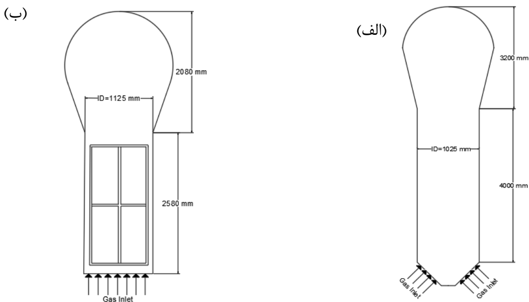
شکل ۱. هندسه ی راکتور های مورد استفاده برای مقایسه هیدرودینامیکی راکتور مورد استفاده در (الف) تکنولوژی بازل (ب) تکنولوژی میتسوئی
