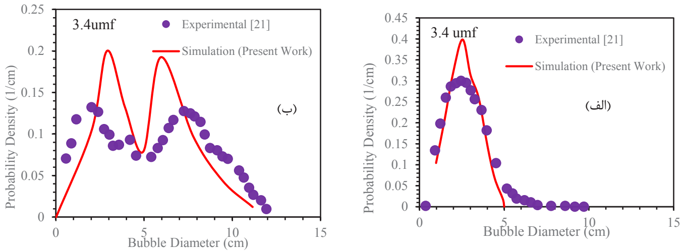
شکل ۵. مقایسه ی توزیع اندازه حبابها در ارتفاع (الف) ۹۰ و (ب) ۲۷۰ میلیمتری از کف بستر و سرعت ۳/۴ برابر حداقل سرعت سیالیت بین داده های شبیه سازی و آزمایشگاهی: ارتفاع راکتور: ۸۰۰ میلیمتر، عرض راکتور: ۱۸۰ میلیمتر، ارتفاع اولیه بستر: ۳۶۰ میلیمتر، قطر ذرات جامد: ۲۵۰ میکرون، دانسیته ذرات جامد: 2500 \text{ kg/m}^3 ، حداقل سرعت سیالیت: 5.24 \text{ cm/s} ، گاز ورودی: هوا. میانگین خطای نسبی شکل الف: ۷ درصد و شکل ب: ۳۸ درصد
