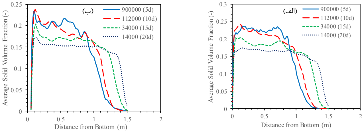
شکل ۳. مقدار میانگین زمانی کسر حجمی ذرات جامد (زمان ۱۰ تا ۳۰ ثانیه) در جهت محوری راکتور (الف) در مرکز و (ب) وسط حد واصل مرکز و دیوار راکتور مورد استفاده برای عملیات استقلال از شبکه (ارتفاع: ۲۵۰۰ میلیمتر، قطر: ۵۱۰ میلیمتر، قطر ذرات جامد: ۱۶۸۵ میکرون، دانسیته ذرات جامد: 918 \text{ kg/m}^3 ، سرعت گاز ورودی: 0.61 \text{ m/s} ، ویسکوزیته گاز ورودی: 1.185 \times 10^{-5} \text{ Pa.s} )
