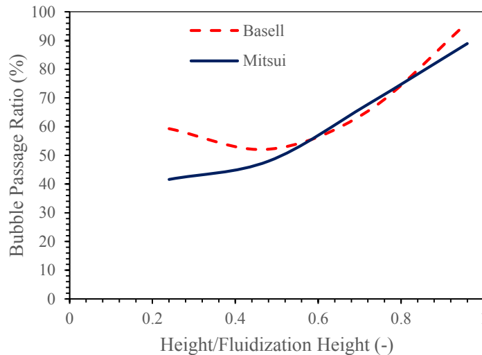
شکل ۱۰. بررسی درصد عبور جریان گازی از جریان حبابی در راکتورهای بازل و میتسویی
