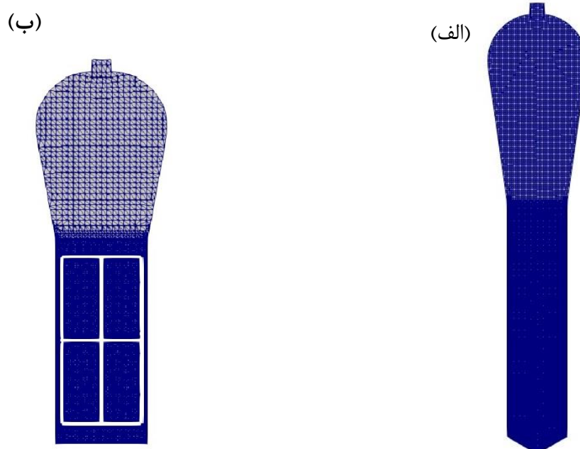
شکل ۲. برشی از شبکه تولید شده برای دو راکتور صنعتی شبیه سازی شده: (الف) تکنولوژی بازل (ب) تکنولوژی میتسوئی
