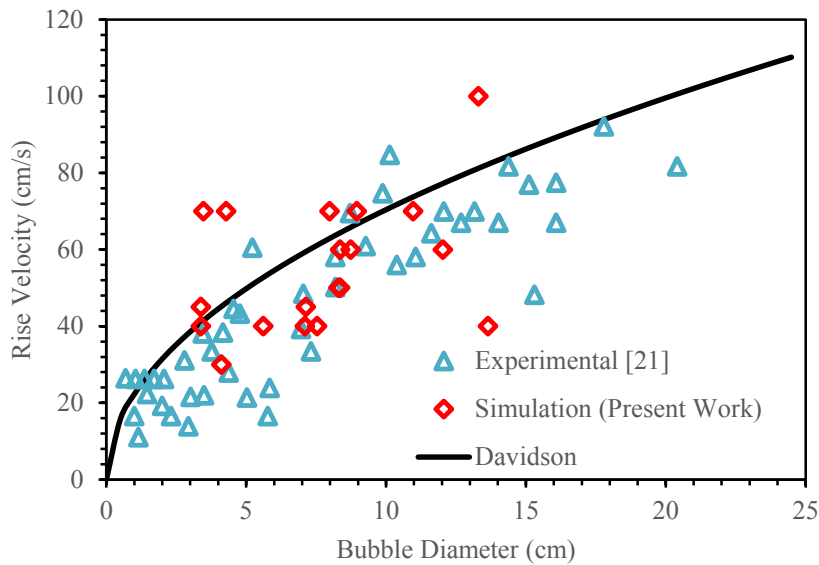
شکل ۴. مقایسه ی توزیع سرعت بالا رفتن حبابها با قطر متغیر حاصل از شبیه سازی و داده های آزمایشگاهی [۲۱] و رابطه ی داویدسون و هریسون [۲۴]: ارتفاع راکتور: ۸۰۰ میلیمتر، عرض راکتور: ۱۸۰ میلیمتر، ارتفاع اولیه بستر: ۳۶۰ میلیمتر، قطر ذرات جامد: ۲۵۰ میکرون، دانسیته ذرات جامد: ۲۵۰۰ kg/m ۳ ، حداقل سرعت سیالیت: ۵/۲۴ cm/s، گاز ورودی: هوا
