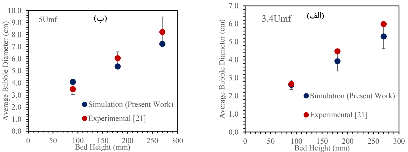
شکل ۷. میانگین قطر حبابها در ارتفاعات ۹۰، ۱۸۰ و ۲۷۰ میلیمتری از کف بستر و سرعت (الف) ۳/۴ و (ب) ۵ برابر حداقل سرعت سیالیت بین داده های شبیه سازی و آزمایشگاهی [۲۱]: ارتفاع راکتور: ۸۰۰ میلیمتر، عرض راکتور: ۱۸۰ میلیمتر، ارتفاع اولیه بستر: ۳۶۰ میلیمتر، قطر ذرات جامد: ۲۵۰ میکرون، دانسیته ذرات جامد: ۲۵۰۰ kg/m ۳ ، حداقل سرعت سیالیت: ۵/۲۴ cm/s، گاز ورودی: هوا
