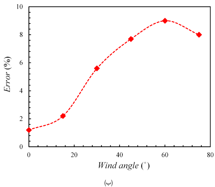
شکل ۴. الف) مقایسه نتایج بدست آمده در زاویه‌های متفاوت وزش باد بین داده‌های تجربی اهبا و همکاران [۲۸] و نتایج کار عددی حاضر و ب) درصد خطای کار عددی حاضر در مقایسه با کار تجربی مرجع [۲۸]
