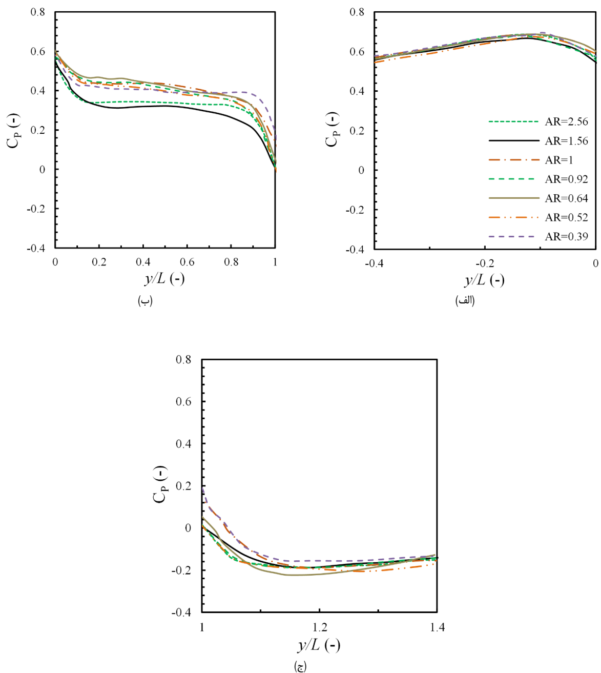
شکل ۱۳. ضریب فشار بدست آمده مربوط به نقاط موجود بر خط اتصال مراکز ورودی و خروجی ساختمان واقع در صفحه میانی ساختمان در مطالعه عددی حاضر برای مدل‌های با ابعاد پنجره متفاوت در سه ناحیه مختلف، (الف) جلوی ساختمان، (ب) نواحی داخلی ساختمان و (ج) پشت ساختمان
