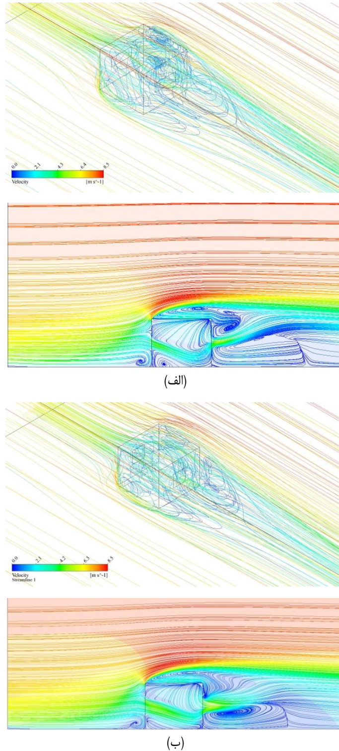
شکل ۱۴. کانتور سه بعدی و دو بعدی خطوط جریان در داخل و خارج ساختمان، (الف) ساختمان با نرخ تناسب پنجره برابر ۰/۳۹ و (ب) ساختمان با نرخ تناسب پنجره برابر ۱
