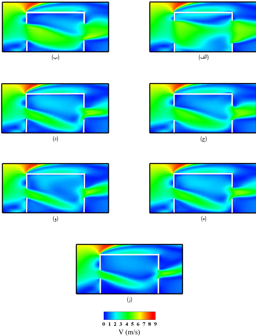
شکل ۱۰. کانتور تغییرات سرعت برای مدل‌های با مقادیر متفاوت نرخ تناسب (الف) AR=2/56 ، (ب) AR=1/56 ، (ج) AR=1 ، (د) AR=0/92 ، (ه) AR=0/64 ، (و) AR=0/52 و (ز) AR=0/39
