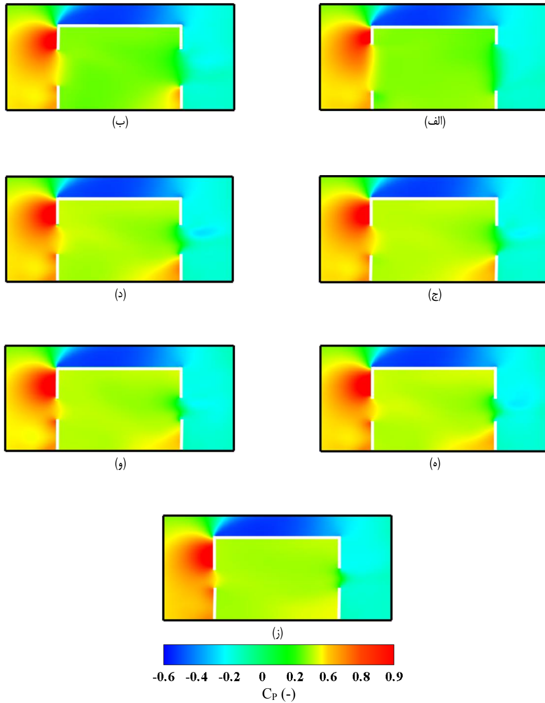
شکل ۱۱. کانتور ضریب فشار در صفحه عمودی میانی ساختمان برای مدل‌های با مقادیر متفاوت نرخ تناسب (الف) AR=2/56 ، (ب) AR=1/56 ، (ج) AR=1 ، (د) AR=0/92 ، (ه) AR=0/64 ، (و) AR=0/52 و (ز) AR=0/39
