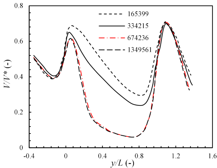
شکل ۵. بررسی استقلال از مش حل عددی مطالعه حاضر برای شبکه‌های محاسباتی با تعداد سلول ۱۶۵۳۹۹، ۳۳۴۲۱۵، ۶۷۴۲۳۶ و ۱۳۴۹۵۶۱ مربوط به پروفیل سرعت نقاط موجود بر خط اتصال مراکز ورودی و خروجی ساختمان واقع در صفحه میانی ساختمان
