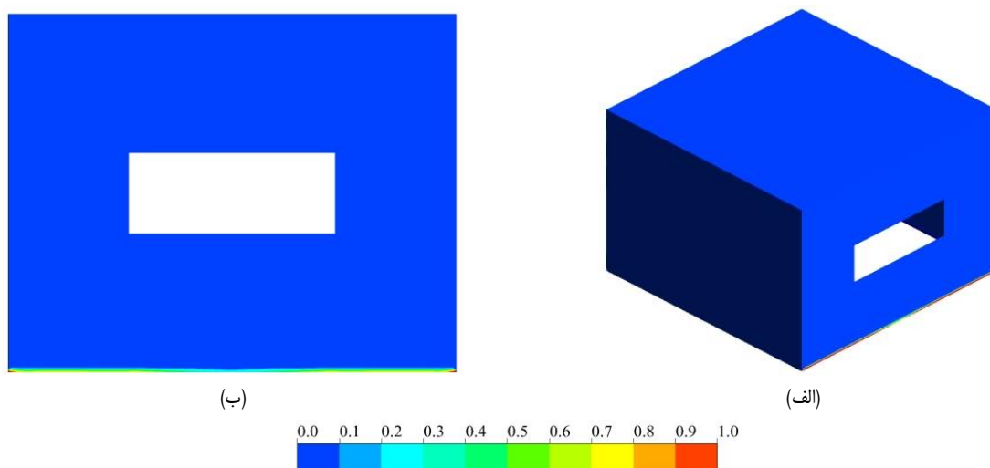
شکل ۶. کانتور توزیع y^+ در مجاورت دیواره‌های ساختمان در مدل مرجع شبیه‌سازی شده، (الف) نمایش توزیع مذکور در دیواره‌های ساختمان به صورت سه بعدی و (ب) نمایش توزیع مذکور در دیواره پشت به باد به صورت دو بعدی
