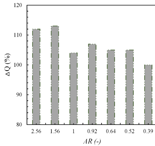
شکل ۷. درصد افزایش نرخ دبی حجمی برای مدل‌های با ابعاد پنجره متفاوت در زاویه وزش صفر درجه باد نسبت به مدل مرجع
