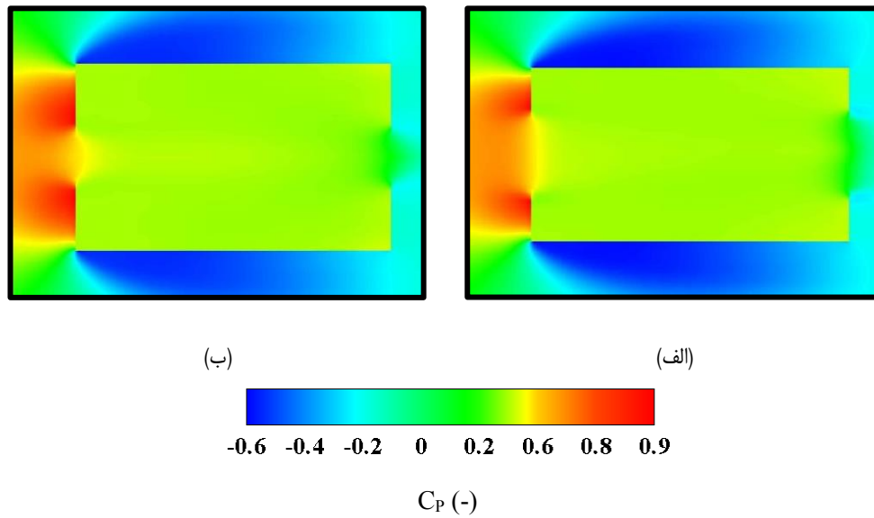
شکل ۱۲. کانتور ضریب فشار در صفحه میانی افقی ساختمان برای مدل‌های با مقادیر متفاوت نرخ تناسب (الف) AR=0.39 و (ب) AR=1
