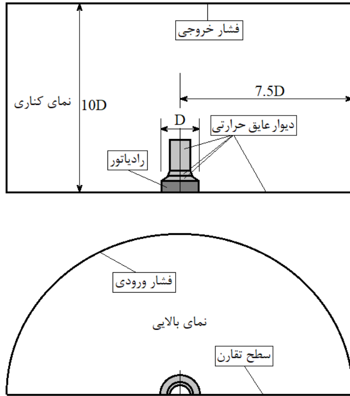
شکل ۳. ابعاد میدان جریان و شرایط مرزی در مدل عددی برای شرایط طراحی.
