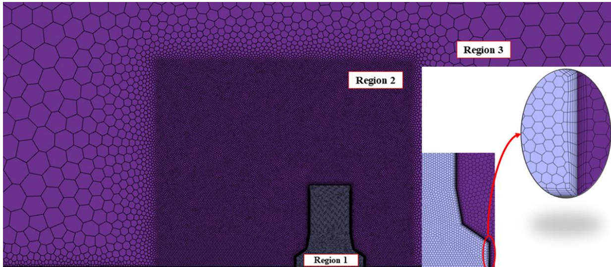
شکل ۵. نمایش جزئیات شبکه با المان‌های چندوجهی در صفحه منطبق بر صفحه تقارن برج خنک‌کن.
