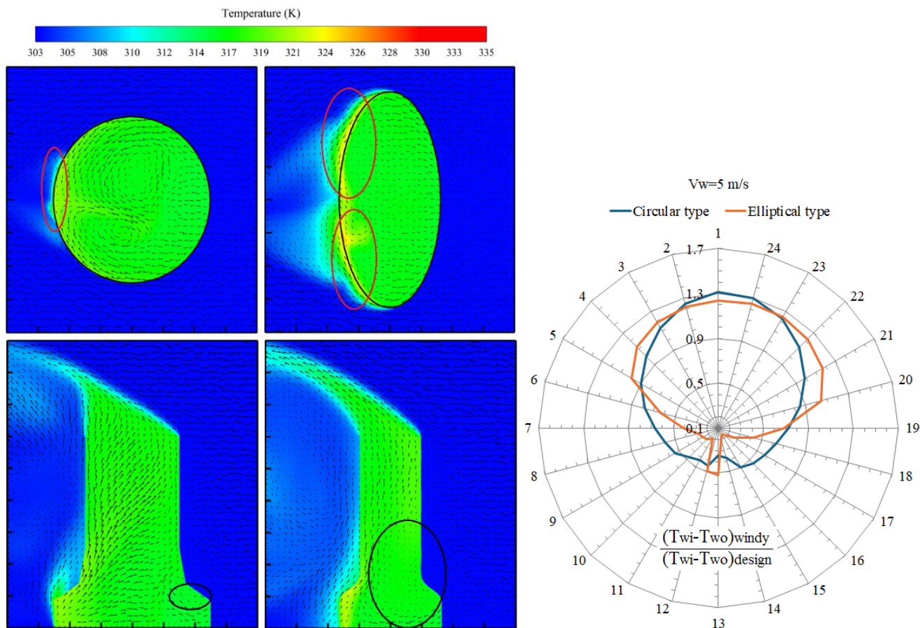
شکل ۹. طیف دما و بردارهای سرعت، و توزیع دمای بی‌بُعد آب خروجی از رادیاتورهای در سرعت باد ۵ متر بر ثانیه.
