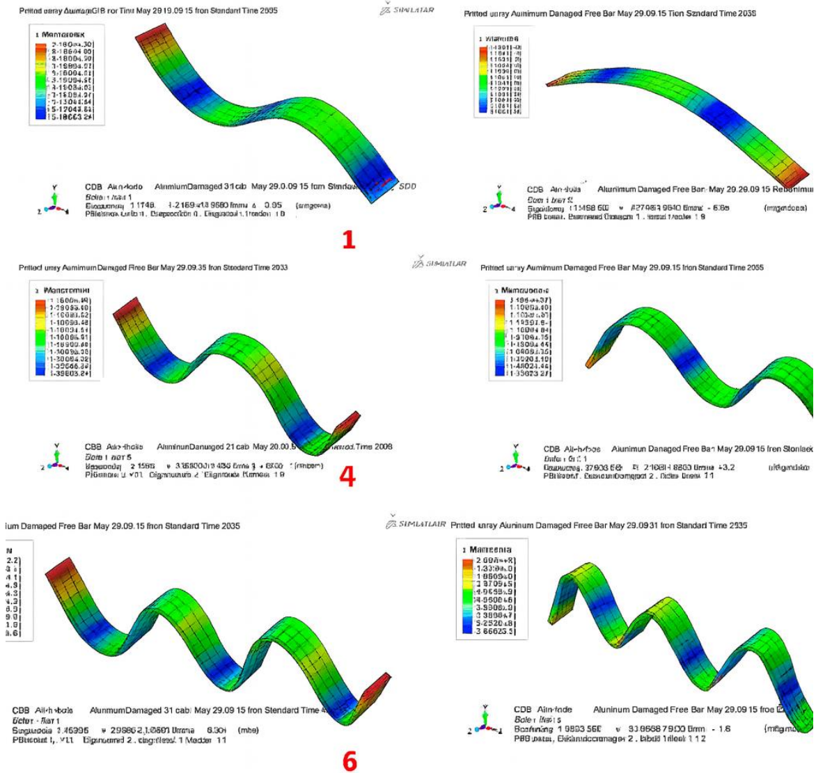
شکل ۱۶. شکل‌مادهای خمشی اول تا ششم تیر آسیب دیده استخراج شده از تحلیل آباکوس (ترک در وسط تیر با عمق ۵۰ درصد)
