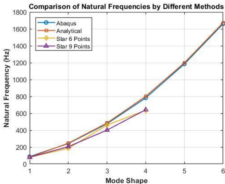
شکل ۲۲. نمودار مقایسه نتایج بدست آمده.
