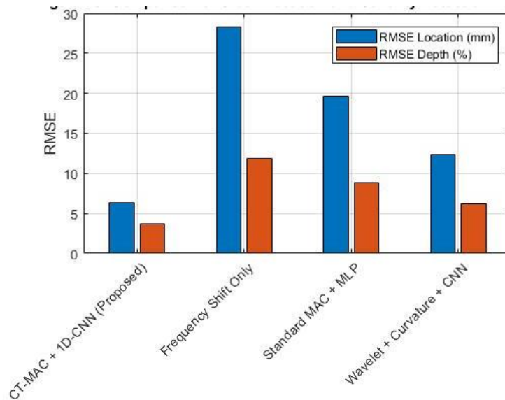
شکل ۲۰. مقایسه دقت روش پیشنهادی معیار اطمینان مودال بهبود یافته با کانتورلت با روش‌های مرسوم (ریشه میانگین مربعات خطا محل و عمق ترک).
