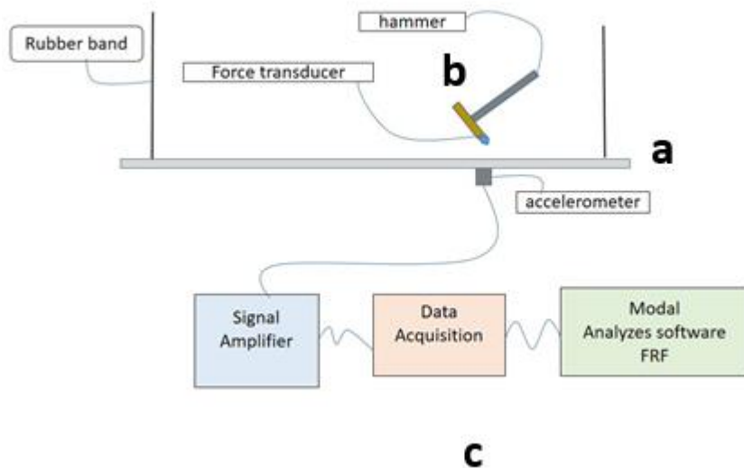
شکل ۱. ستاپ آزمایش مودال تجربی تیر آلومینیومی دوسر آزاد: (a) نمای کلی تیر معلق با طناب‌های الاستیک برای شبیه‌سازی شرایط مرزی آزاد-آزاد، (b) موقعیت چکش ضربه‌ای کالیبره‌شده و شتاب‌سنج تک‌محوره چسبانده‌شده با موم در نقطه مرجع، (c) اتصال به آمپلی‌فایر و سیستم اکتساب داده.
