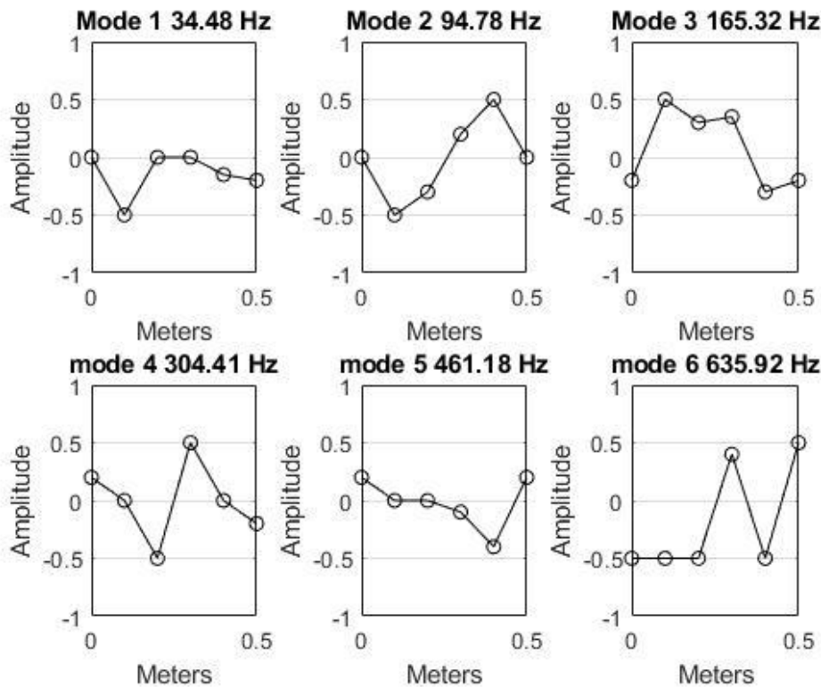
شکل ۱۲. شکل‌مادهای خمشی اول تا ششم تیر سالم استخراج‌شده از تست مودال.
