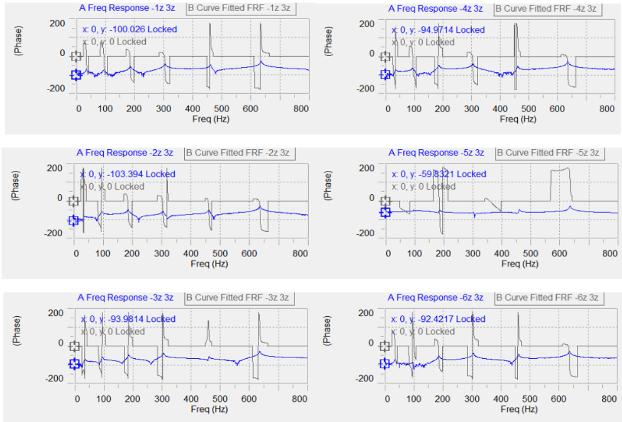
شکل ۷. نمودار فاز بر اساس نقاط تحریک استخراج شده از نرم‌افزار استار.
