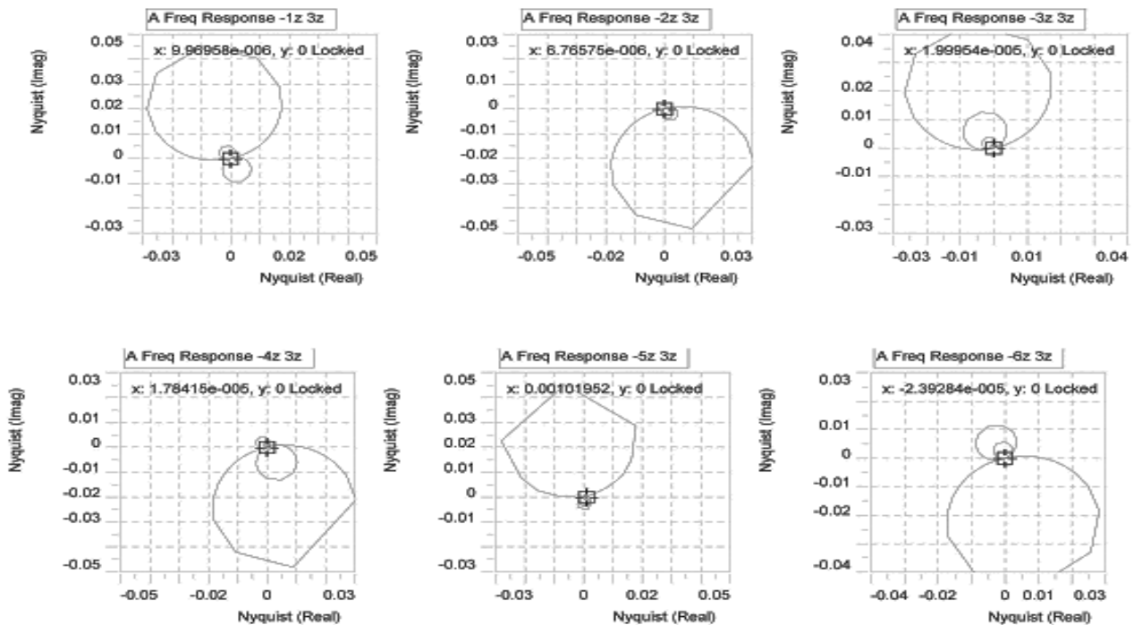
شکل ۱۱. نمودار نایکوست برای نقاط مختلف تحریک استخراج شده از نرم افزار استار
