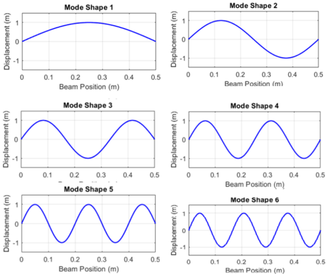
شکل ۳. شکل‌مودهای خمشی اول تا ششم تیر سالم استخراج‌شده از حل تحلیلی درمطلب نرمال‌سازی نسبت به بیشینه جابجایی.
