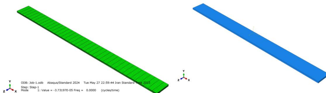
شکل ۲. تعریف هندسه و مش بندی تیر آلومینیومی در نرم افزار آباکوس.
