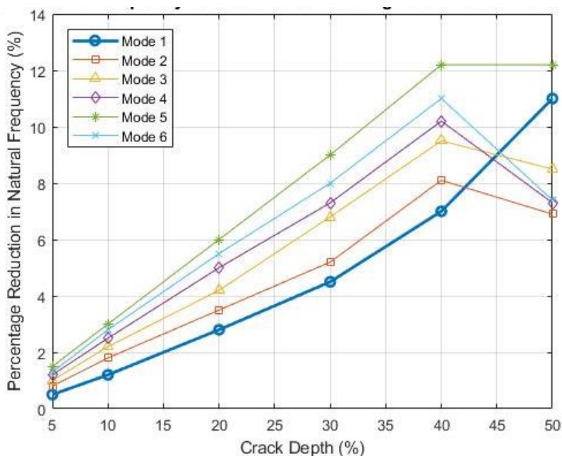
شکل ۲۱. درصد کاهش فرکانس طبیعی شش مود خمشی در حضور ترک عرضی با عمق‌های مختلف (۵ درصد تا ۵۰ درصد).
