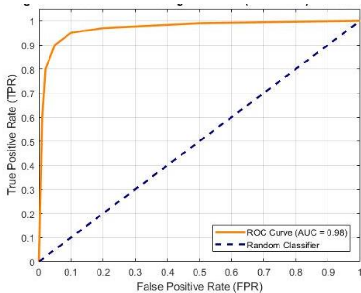
شکل ۱۹. منحنی مشخصه عملکرد گیرنده برای تشخیص دو کلاس وجود یا عدم وجود آسیب با روش معیار اطمینان مودال بهبود یافته با کانتورلت (AUC = 0.98) در حضور نویز ۵ درصد.
