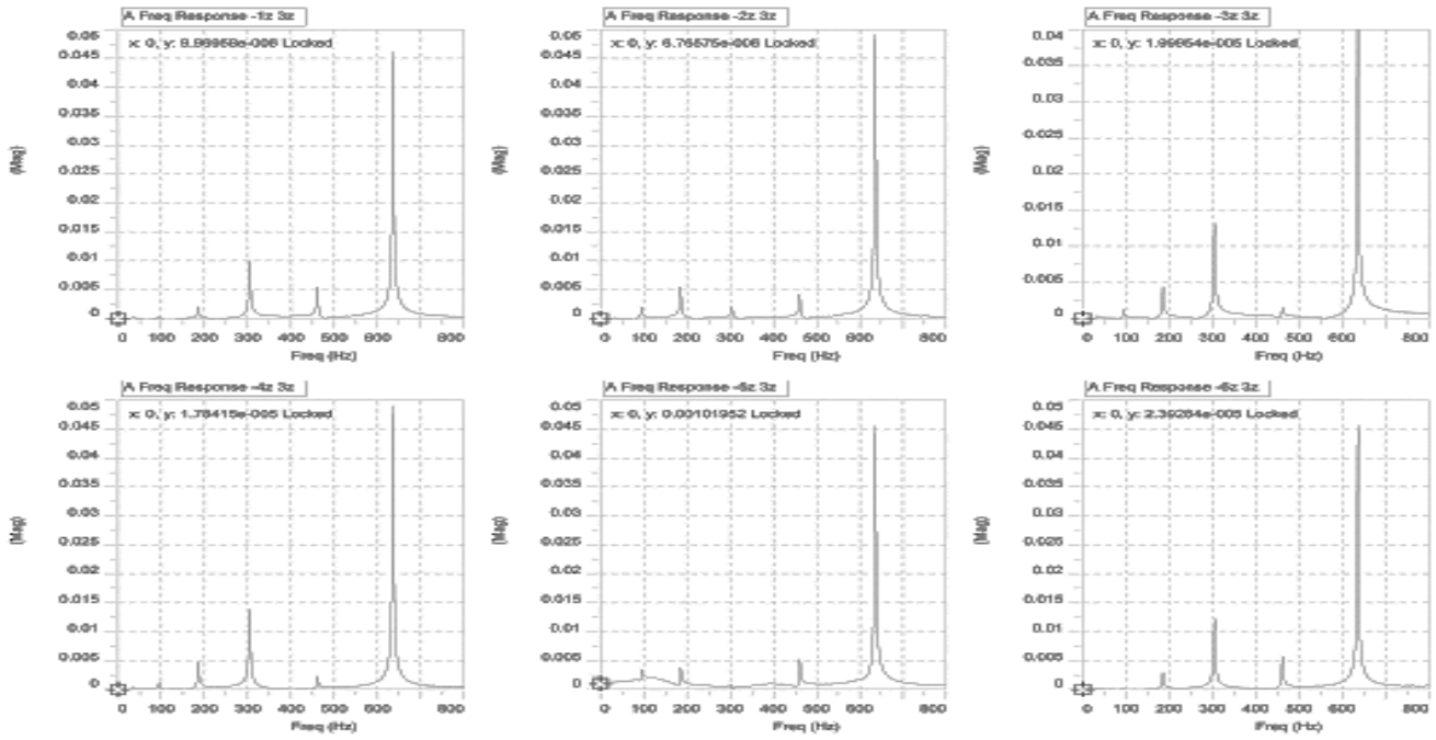
شکل ۸. نمودار تغییرات دامنه در بازه فرکانس در نرم افزار استار برای شش نقطه استخراج شده از نرم افزار استار.
