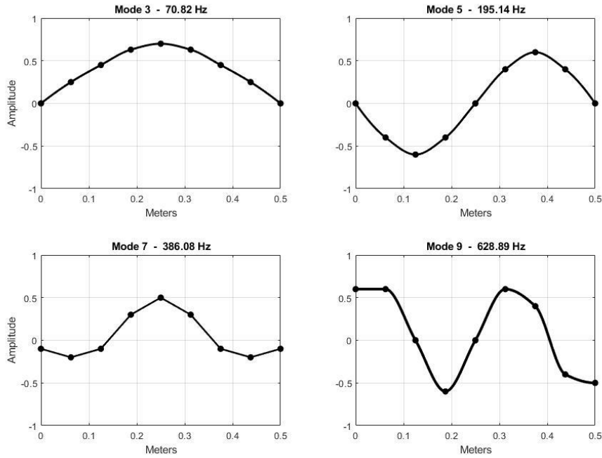
شکل ۱۴. شکل مودهای خمشی اصلی استخراج شده از تست مودال با تحریک ۹ نقطه.
