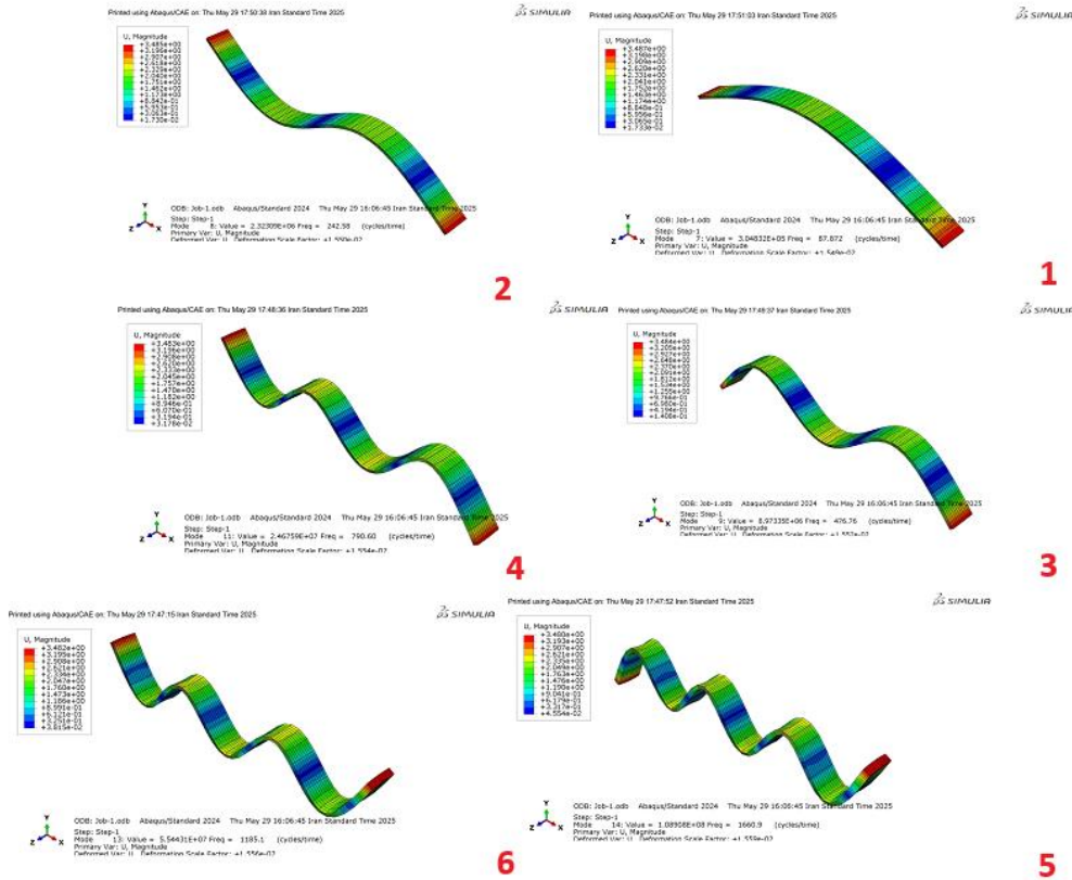
شکل ۱۵. شکل مودهای خمشی اول تا ششم تیر سالم استخراج شده از تحلیل آباکوس.
