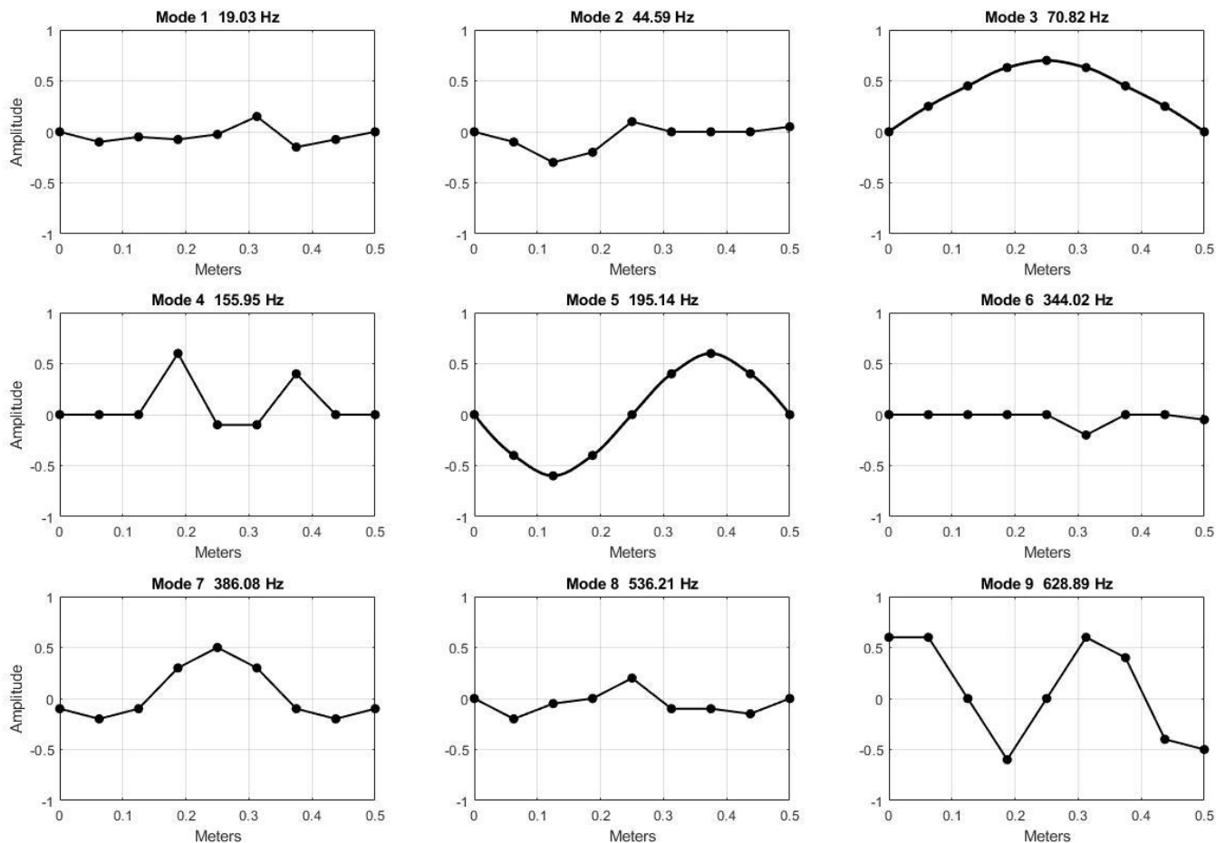
شکل ۱۳. شکل‌مدهای خمشی اول تا نهم تیر سالم استخراج‌شده از تست مودال.
