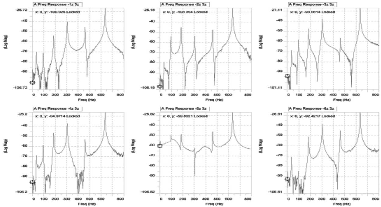
شکل ۱۰. نمودار تابع پاسخ فرکانسی تیر تحریک شده در نرم افزار استار برای شش نقطه استخراج شده از نرم افزار استار.
