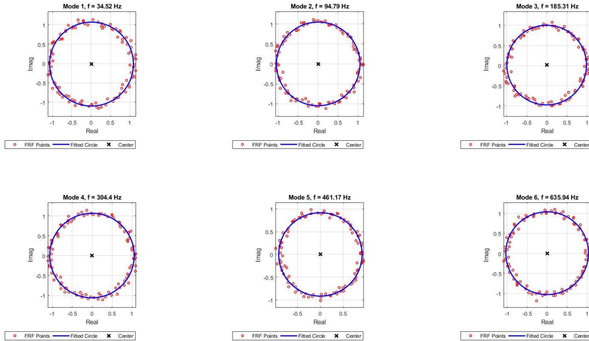
شکل ۴. نمودار سیرکل فیتینگ بر حسب داده‌های خروجی از نرم‌افزار استار.
