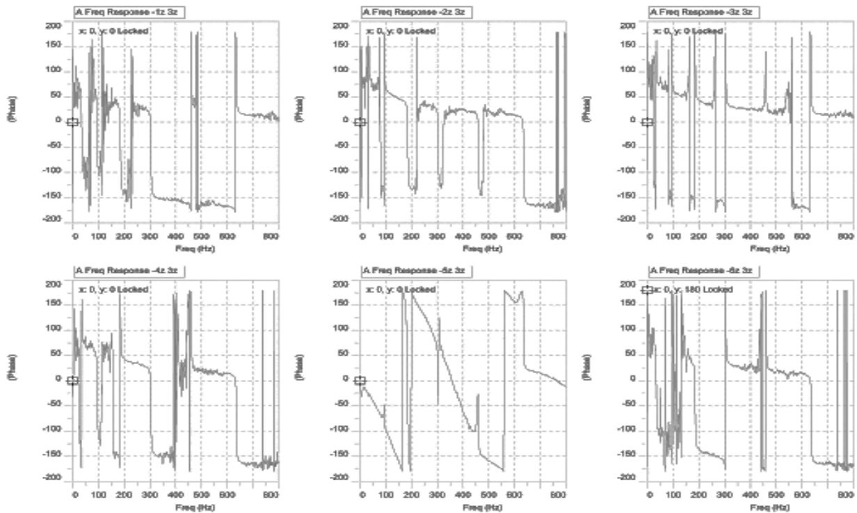
شکل ۹. نمودار تغییرات فاز بر حسب فرکانس در نرم افزار استار برای شش نقطه استخراج شده از نرم افزار استار.
