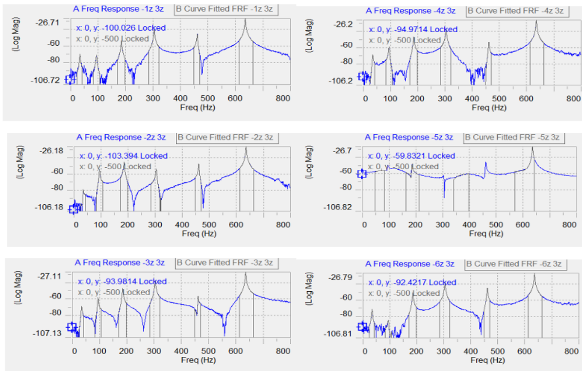
شکل ۶. نمودار تابع پاسخ فرکانسی بر اساس نقاط تحریک استخراج شده از نرم‌افزار استار.
