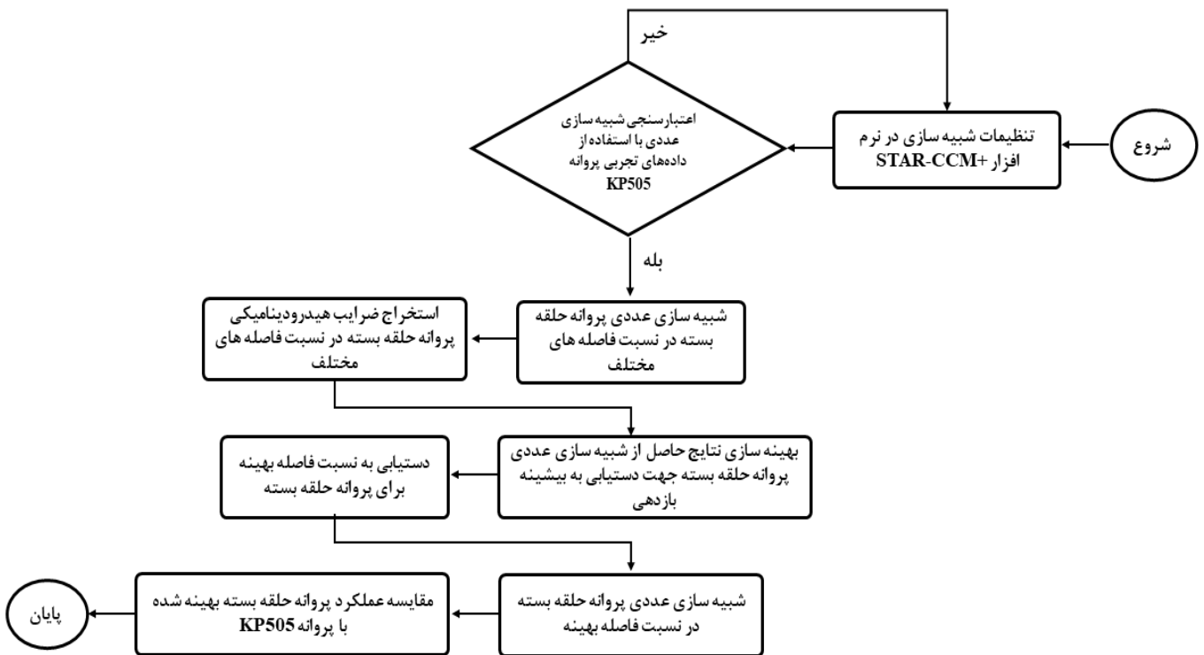
شکل ۲. فلوچارت تعریف مسئله.
