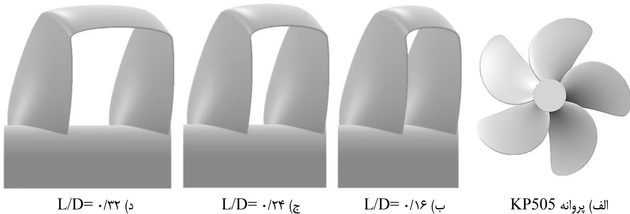
شکل ۴. پروانه‌های شبیه‌سازی شده در پژوهش حاضر.
