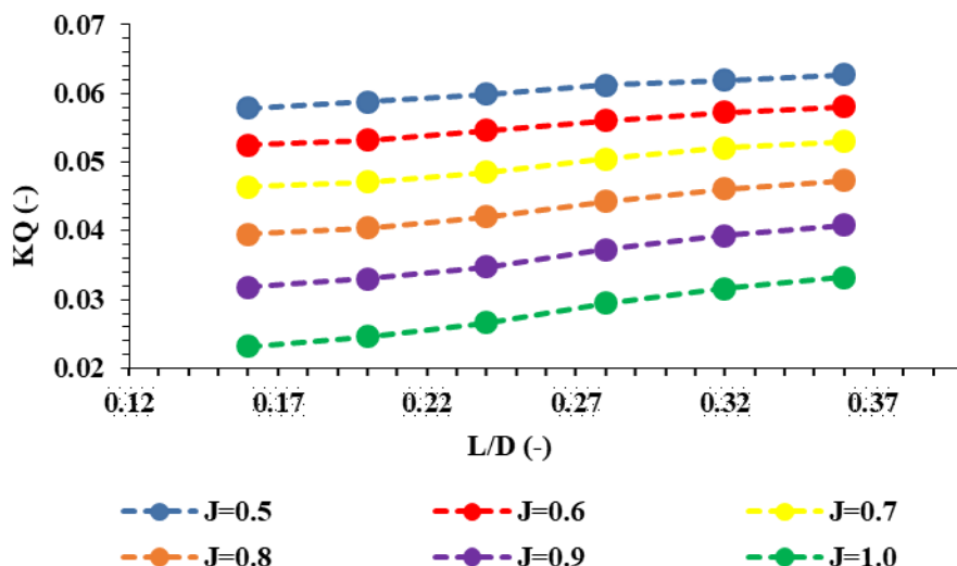
شکل ۱۲. تغییرات ضریب گشتاور بر حسب تغییر نسبت فاصله در ضرایب پیشروی مختلف برای پروانه حلقه بسته.
