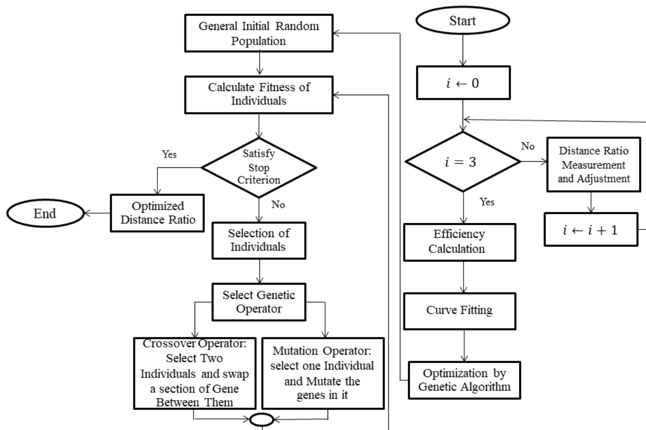
شکل ۸. فلوجارت الگوریتم ژنتیک مورد استفاده در این پژوهش [۲۹].
