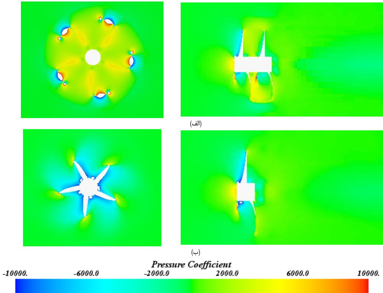
شکل ۱۷. مقایسه تغییرات ضریب فشار در ضریب پیشروی ۰/۸ برای الف) پروانه حلقه بسته بهینه و ب) پروانه KP505.
