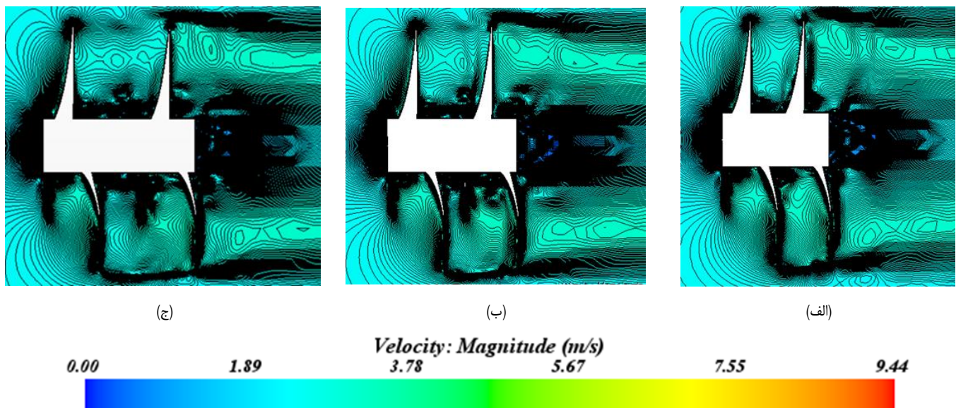
شکل ۱۱. کانتور خطوط تغییرات سرعت در اطراف پروانه در حالت‌های مختلف نسبت فاصله (الف) ۰/۲، (ب) ۰/۲۸ و (ج) ۰/۳۶ در ضریب پیشروی ۰/۸.
