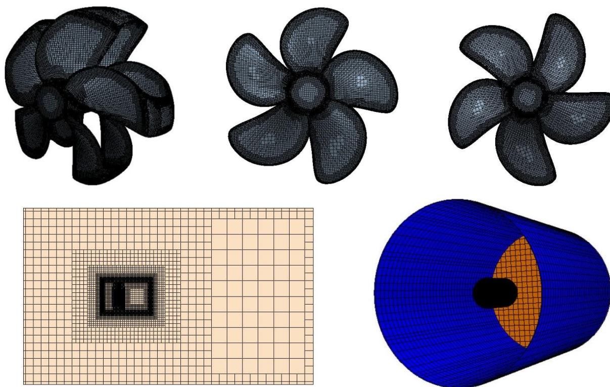
شکل ۵. شبکه‌بندی ایجادشده برای شبیه‌سازی پژوهش حاضر.
