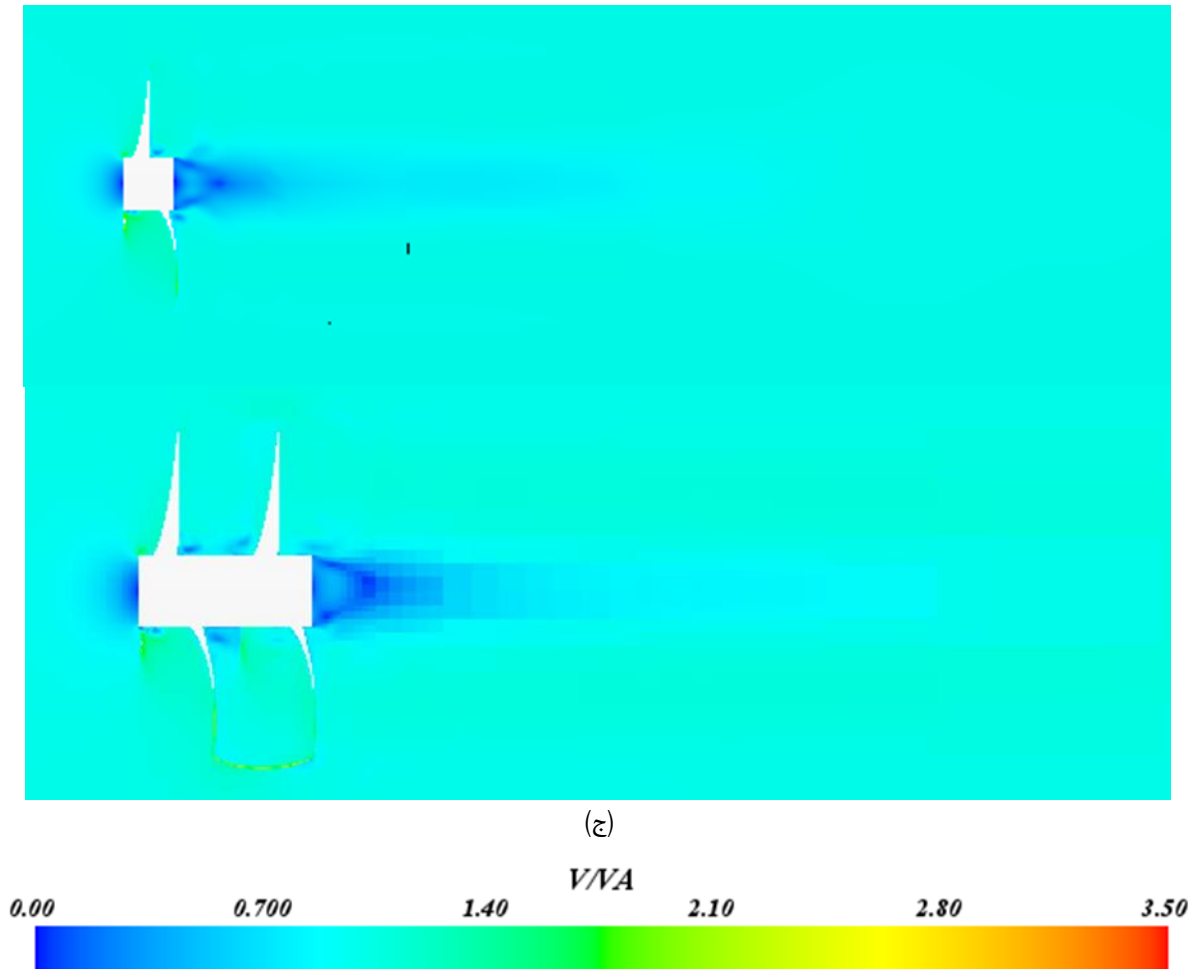
شکل ۱۶. کانتور تغییرات سرعت در راستای جریان اطراف پروانه در ضرایب پیشروی مختلف را برای پروانه حلقه‌بسته بهینه و پروانه KP505 (الف) J=0.5 (ب) J=0.8 و ج) J=1.0 .
