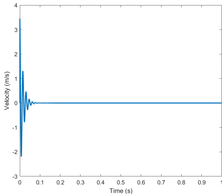
شکل ۲۴. سرعت خطی انتهای تیر هوشمند کامپوزیتی.
