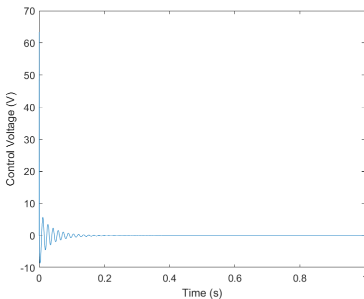
شکل ۲۲. ولتاژ عملگر تیر هوشمند کامپوزیتی.
