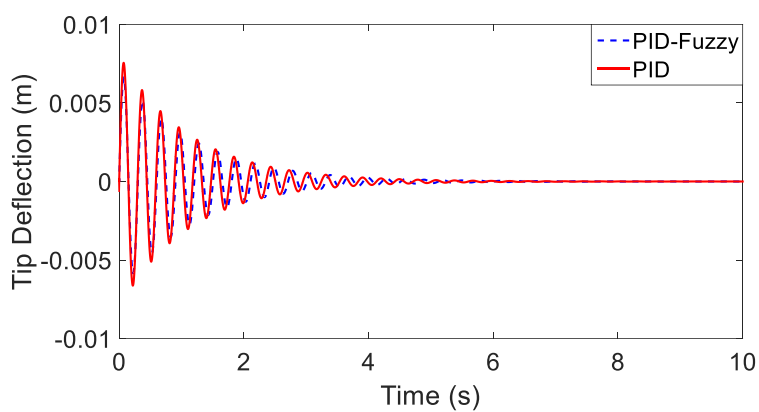
شکل ۱۹. مقایسه کنترل تناسبی-انتگرالی-مشتقی با کنترل فازی در تیر هوشمند اولر.
