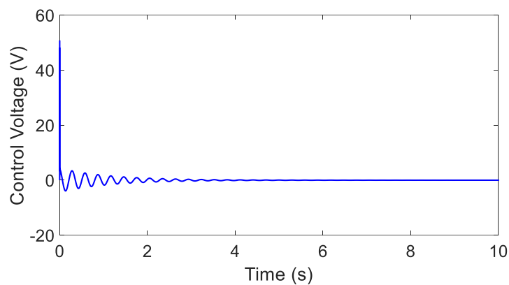
شکل ۱۸. ولتاژ عملکرد تیر هوشمند اولر تحت بار ضربه.
