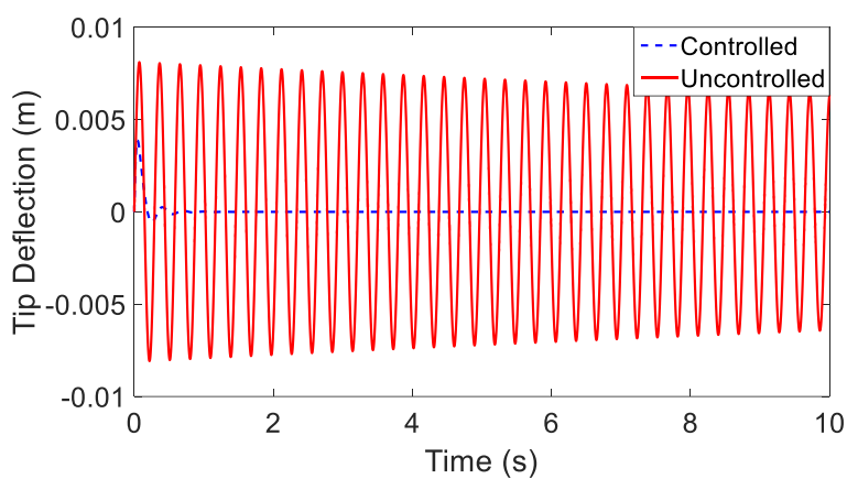
شکل ۱۵. کنترل فازی تیر هوشمند اولر تحت بار ضربه.
