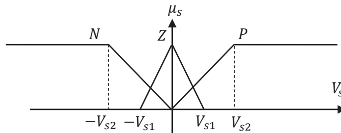
شکل ۶. نمودار تابع تعلق ولتاژ حسگر.
