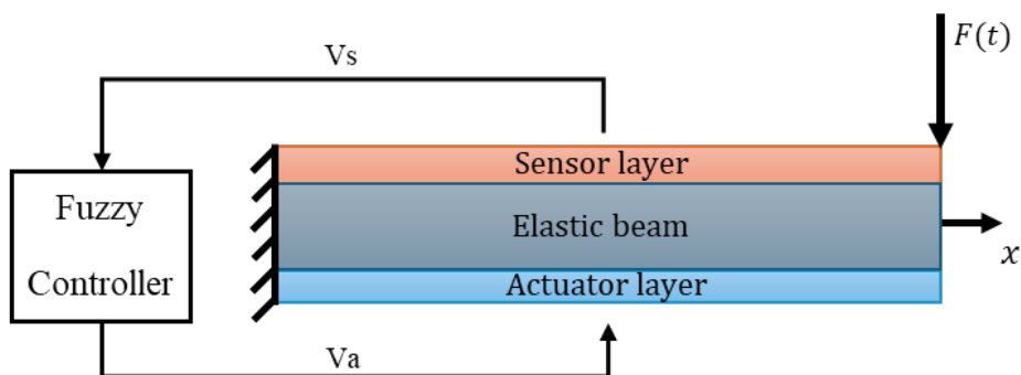
شکل ۵. مدل تیر هوشمند.
