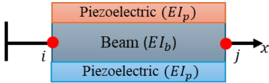
شکل ۲. المان تیر هوشمند اویلر-برنولی.
