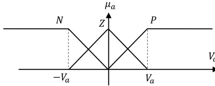
شکل ۷. نمودار تابع تعلق ولتاژ عملگر.
