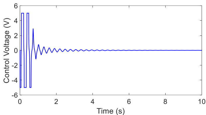
شکل ۱۳. ولتاژ عملکرد تیر هوشمند اولر تحت بار ضربه.
