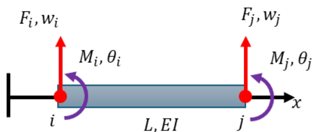
شکل ۱. المان تیر با چهار درجه آزادی.
