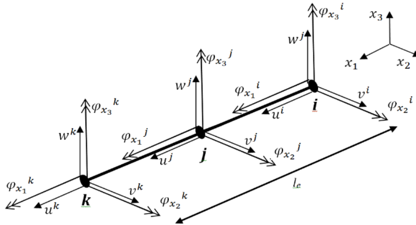
شکل ۴. المان سه‌گره‌ای تیر با ۱۸ درجه آزادی [۱۶].
