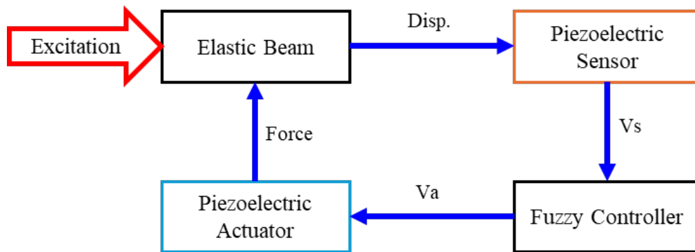
شکل ۸. نمودار کنترلر فازی.
