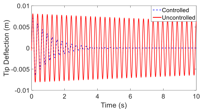
شکل ۱۷. کنترل تناسبی-انتگرالی-مشتقی تیر هوشمند اولر تحت بار ضربه.
