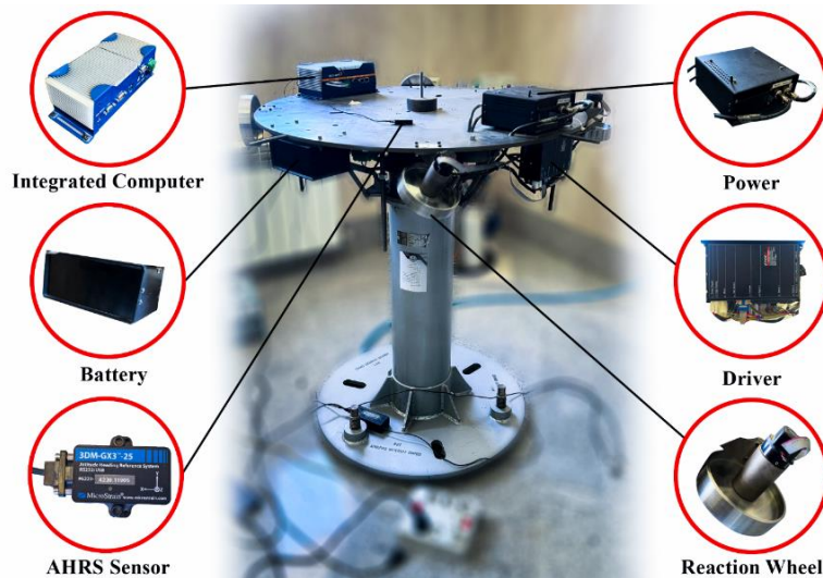
شکل ۱. ساختار کلی شبیه ساز دینامیک وضعیت ماهواره - دانشگاه اصفهان [۱۹].
