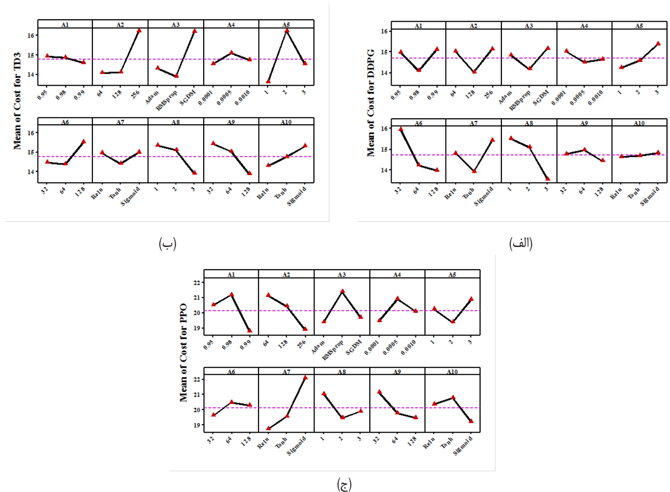
شکل ۳. نتایج بهینه‌سازی فرایارامترهای الگوریتم‌های یادگیری تقویتی عمیق با روش تاگوچی: (الف) DDPG، (ب) TD3، (ج) PPO.
