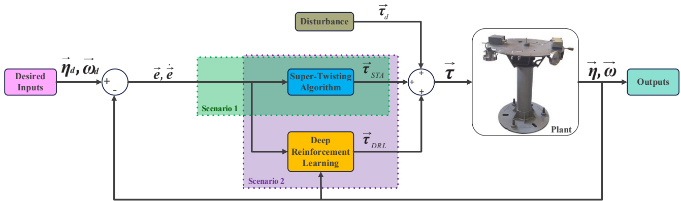
شکل ۲. چارچوب کنترلی برای کنترل وضعیت ماهواره.
