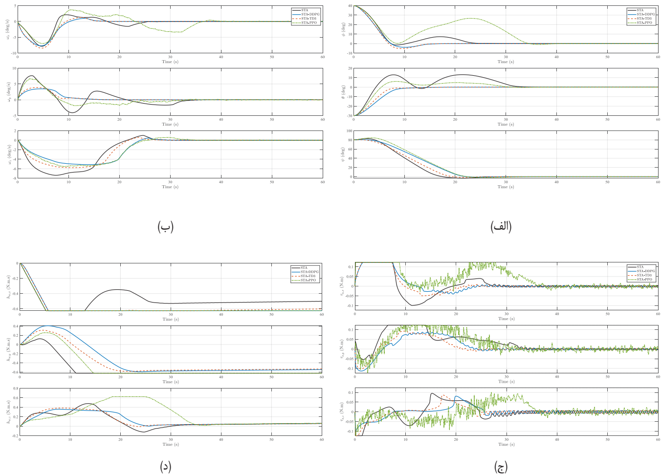
شکل ۶. مقایسه پاسخ‌های شبیه‌سازی چهار روش کنترلی در حضور اغتشاش: (الف) زوایا، (ب) سرعت زاویه‌ای، (ج) ورودی کنترلی، (د) مومنتوم زاویه‌ای.
