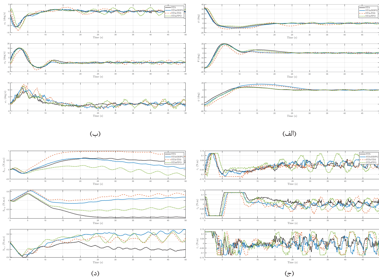
شکل ۸. نتایج پیاده‌سازی مقایسه‌ای چهار روش کنترلی در حضور اغتشاشات ذاتی سکوی آزمایش: (الف) زوایا، (ب) سرعت زاویه‌ای، (ج) ورودی کنترلی، (د) مومنتوم زاویه‌ای.
