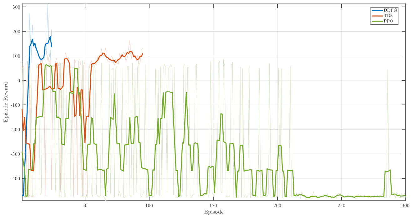
شکل ۴. روند آموزش عامل‌های TD3، DDPG و PPO برای ترکیب نهایی تاگوچی؛ خطوط کم‌رنگ پاداش اپیزودی و خطوط پررنگ میانگین متحرک پاداش با پنجره ۲۰ اپیزودی را نشان می‌دهند.
