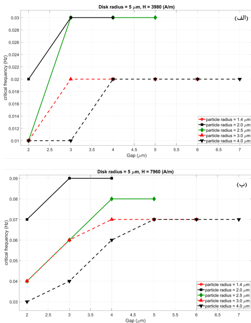
شکل ۶. فرکانس بحرانی ذرات در شکاف‌های مختلف.
