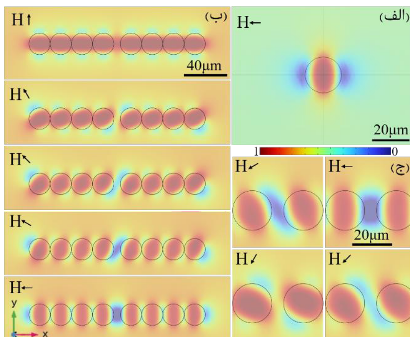
شکل ۳. نتایج شبیه‌سازی توزیع انرژی. (الف) توزیع انرژی مغناطیسی حول یک دیسک مغناطیسی. (ب) توزیع انرژی آرایه‌ای از دیسک‌های مغناطیسی. (ج) نمای بزرگتر توزیع انرژی در فاصله بین دیسک‌ها. فلش‌ها نشان‌دهنده جهت میدان مغناطیسی خارجی می‌باشند. در این شبیه‌سازی انرژی بی بعدسازی شده است.
