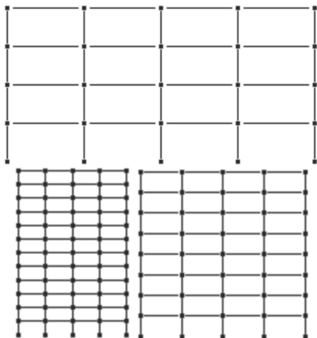
شکل ۳. مدل های غیر خطی ۴، ۸ و ۱۲ طبقه ایجاد شده در Perform-3D.
