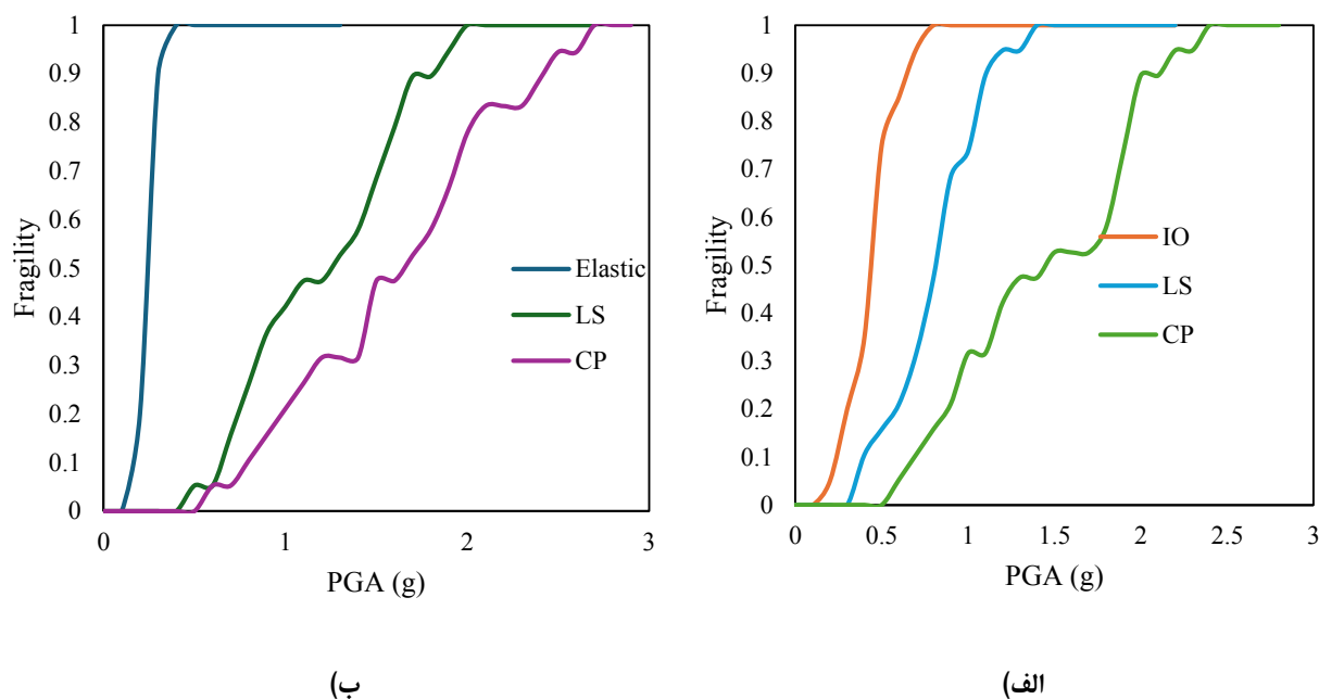
شکل ۱۷. منحنی های شکنندگی سازه دوازده طبقه با روش الف) متداول ب) انرژی.
