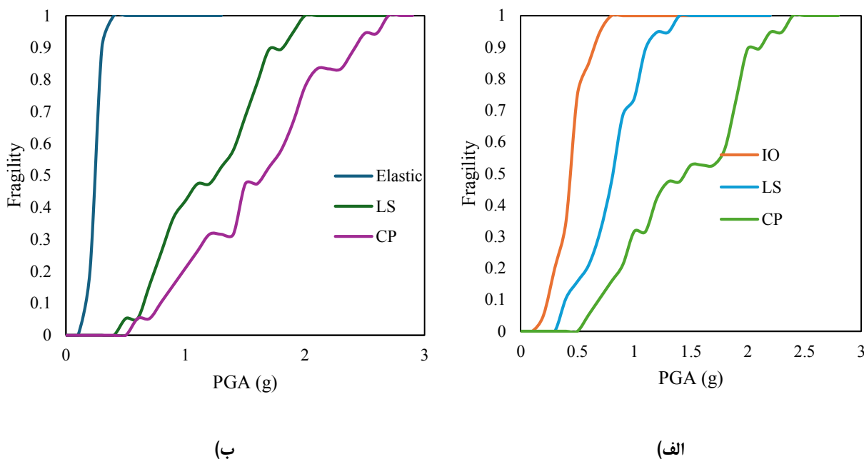
شکل ۱۶. منحنی های شکنندگی سازه هشت طبقه با روش (الف) متداول (ب) انرژی.
