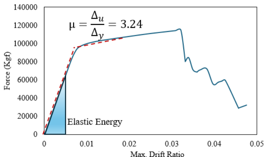
شکل ۱۴. منحنی پوش اور سازه ۱۲ طبقه.
