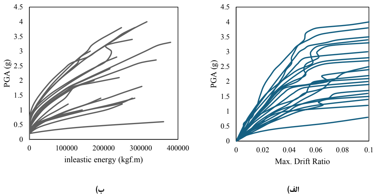
شکل ۱۲. منحنی های IDA سازه ۱۲ طبقه الف) روش متداول ب) روش انرژی.
