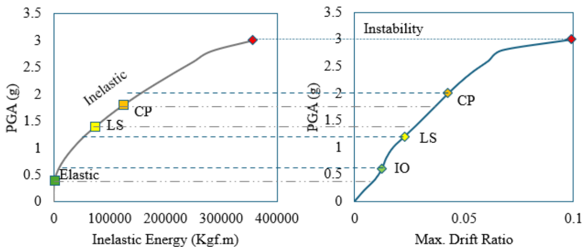
شکل ۱۳. مقایسه منحنی IDA در دو روش متداول و انرژی.
