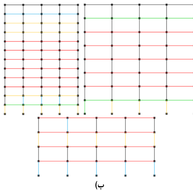
شکل ۶. دوران مفاصل پلاستیک در سطح LS در سازه ها تحت رکورد زلزله GAZLI در بیشینه شتاب الف) ۱/۶ ب) ۱/۸ g.
