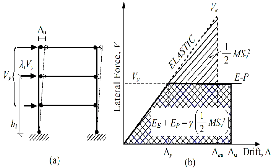
شکل ۴. مفهوم انرژی ورودی طرح، ضریب اصلاح انرژی، انرژی الاستیک و انرژی پلاستیک در سازه.
