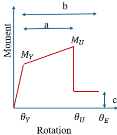
شکل ۲. مدل رفتاری لنگر-دوران برای مدلسازی غیرخطی تیرها.
