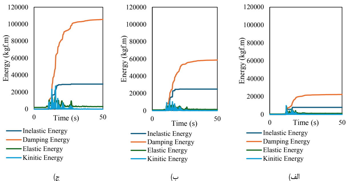
شکل ۸. منحنی های تاریخچه زمانی انرژی های درونی سازه تحت رکورد زلزله ایپریال ولی با بیشینه شتاب 0.6g (الف) سازه ۴ (ب) سازه ۸ (ج) سازه ۱۲ طبقه.
