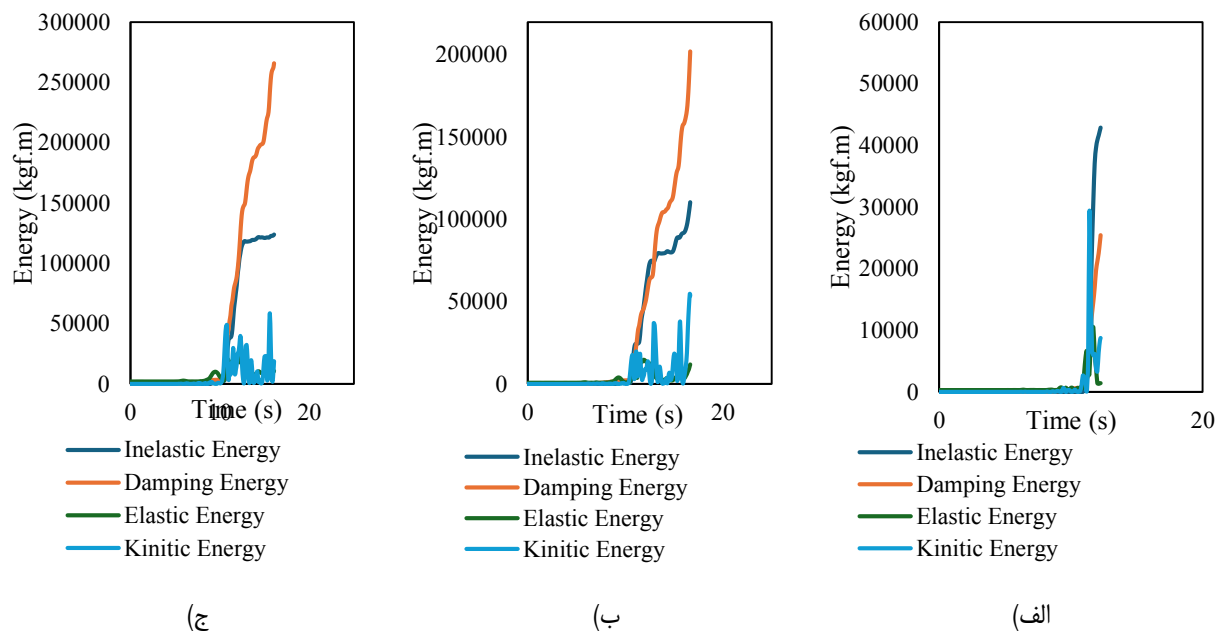
شکل ۹. منحنی های تاریخچه زمانی انرژی های درونی سازه تحت رکورد زلزله ایپریال ولی با بیشینه شتاب g/1.4 (الف) سازه ۴ (ب) سازه ۸ و (ج) سازه ۱۲ طبقه.
