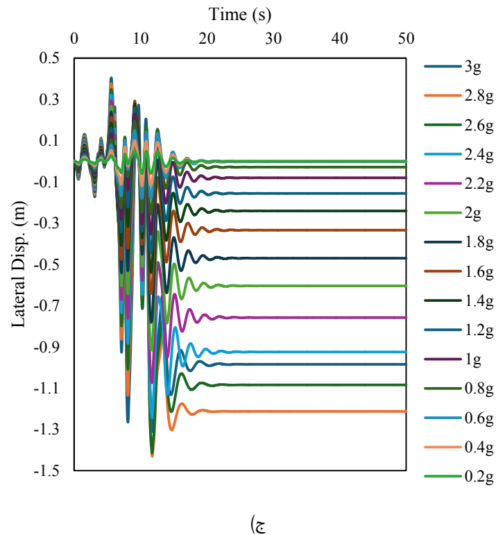
شکل ۵. منحنی تاریخچه زمانی جابجایی افقی بام در زلزله GAZLI در بیشینه شتاب های مختلف در سازه ی الف (۴ ب) ۸ ج) ۱۲ طبقه.
