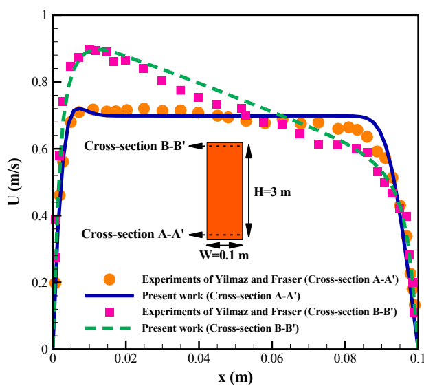
(الف) توزیع سرعت
