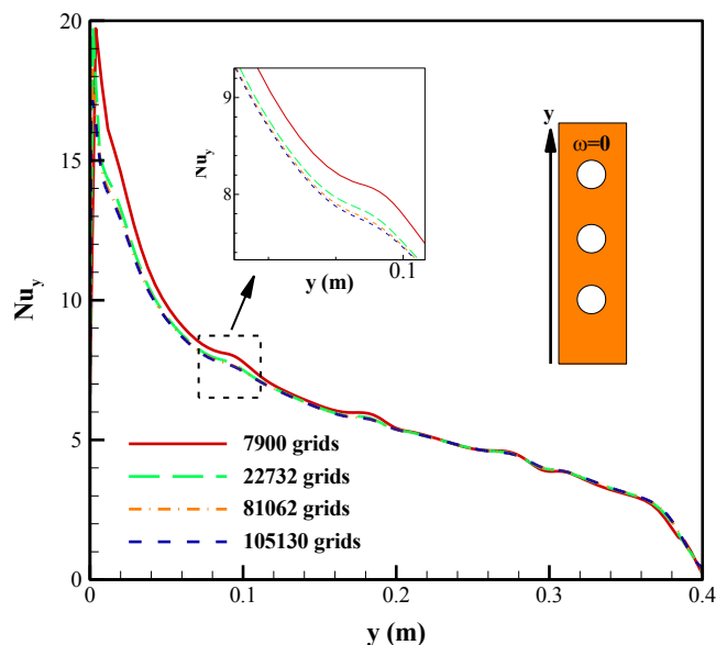
شکل ۳. استقلال از شبکه برای پیکربندی ۲ برای شبکه‌های مختلف (Ra=5 \times 10^5, \omega=0) .
