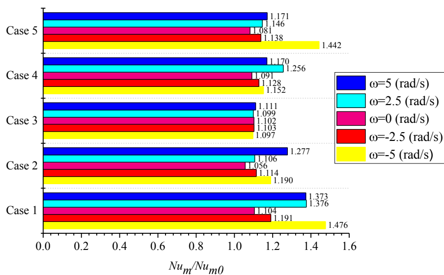
شکل ۸. نسبت عدد ناسلت متوسط محفظه برای پیکربندی‌های مختلف بر حسب سرعت چرخشی متفاوت استوانه‌های چرخان ( Ra=5 \times 10^5 ).
