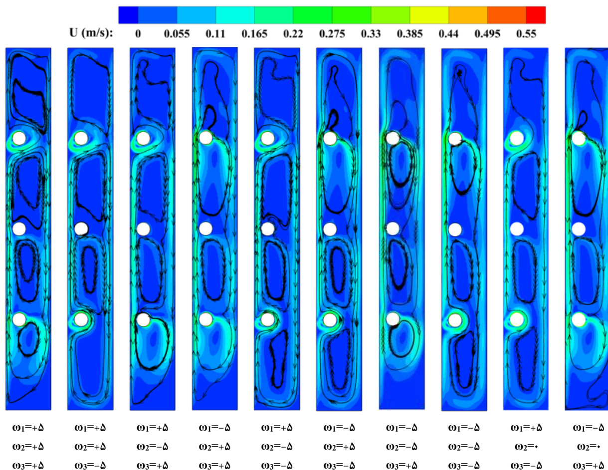
شکل ۱۱. کانتور سرعت و خطوط جریان برای پیکربندی ۱ به ازای چرخش متفاوت هر استوانه ( Ra=5 \times 10^5 , |\omega|=5 ).
