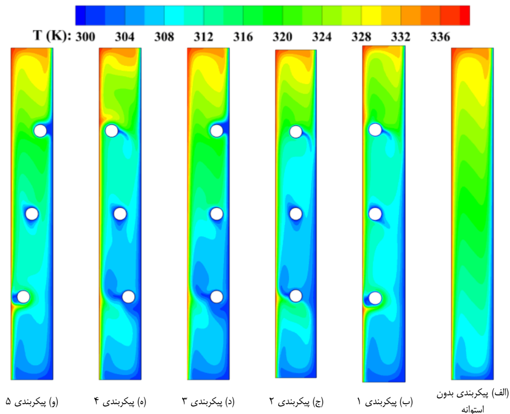
شکل ۷. توزیع دما برای پیکربندی‌های مختلف ( Ra=5 \times 10^5 , \omega=-5 ).
