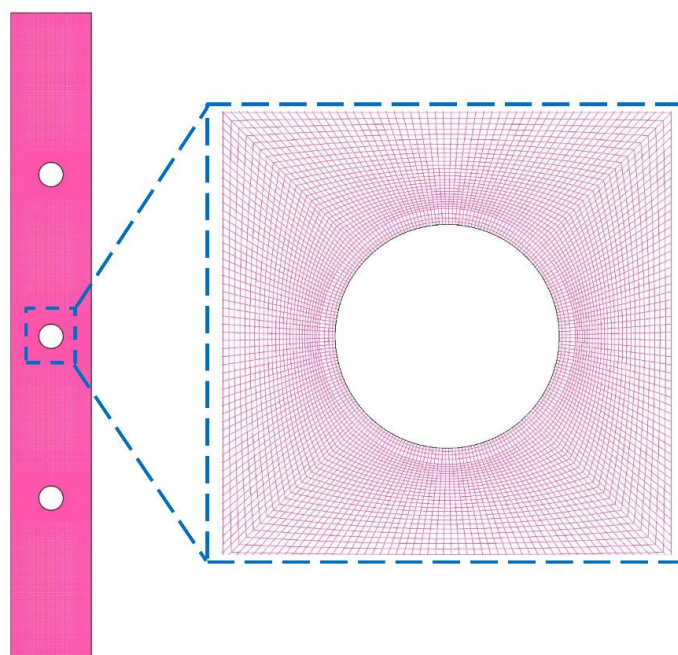
شکل ۲. نمایشی از شبکه محاسباتی برای پیکربندی ۲.
