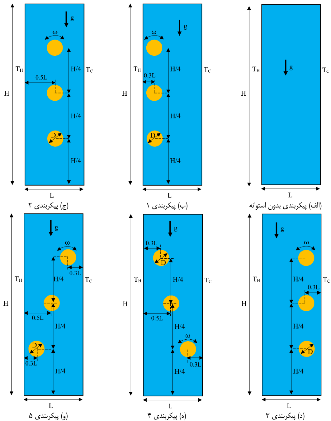
شکل ۱. نمایی شماتیک از هندسه محاسباتی.
