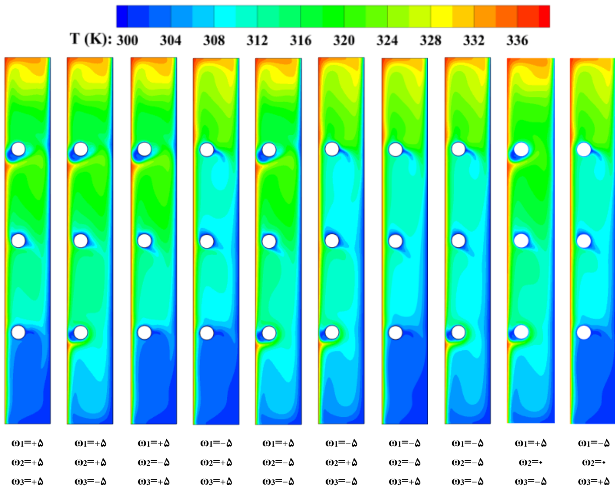
شکل ۱۲. کانتور دما برای پیکربندی ۱ به ازای چرخش متفاوت هر استوانه ( Ra=5 \times 10^5 , |\omega|=5 ).
