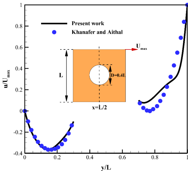
شکل ۵. مقایسه توزیع سرعت افقی با نتایج خانافر و آیدال [۱۴] در مقطع x/L=0.5 به ازای Re=100 و \omega=-0.5 .
