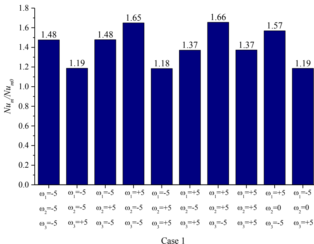
شکل ۱۳. نسبت عدد ناسلت متوسط محفظه برای پیکربندی ۱ به ازای چرخش متفاوت هر استوانه ( Ra=5 \times 10^5 , |\omega|=5 ).
