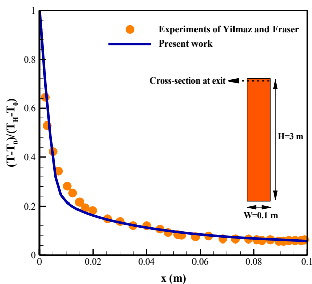
(ب) توزیع دمای بی‌بعد
