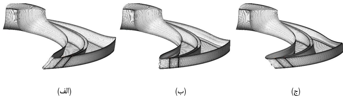
شکل ۶. شبکه بندی کانال بین دو پره برای سه حالت طراحی پره (الف) زاویه ۴۵°، (ب) ۰° و (ج) ۴۵-° درجه).
