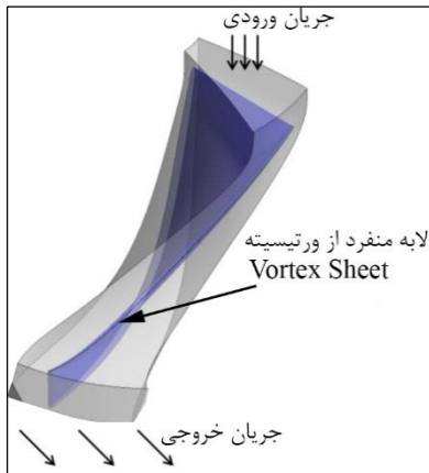
شکل ۱. یک ورقه منفرد از ورتیسیت به جهت مدل سازی پره.
