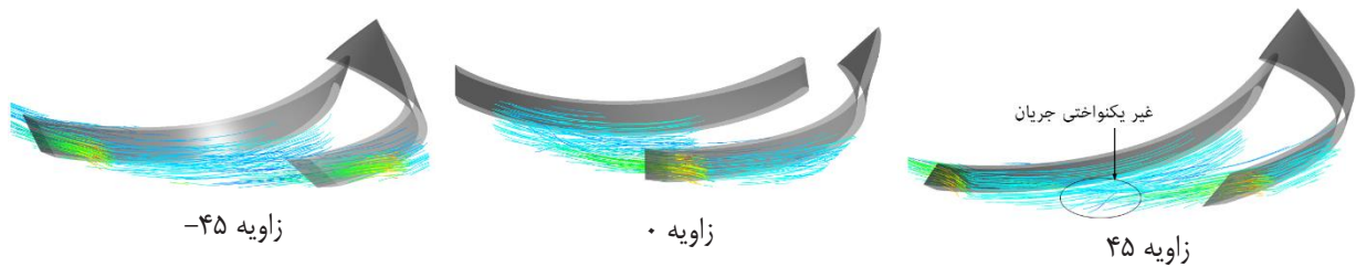
شکل ۱۱. خطوط جریان در مقطع خروجی پروانه در سه حالت زاویه ۴۵+ و ۴۵-.
