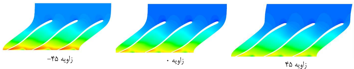
شکل ۱۲. کانتور فشار استاتیکی در پروانه در سه حالت زاویه ۴۵+ و ۴۵-.
