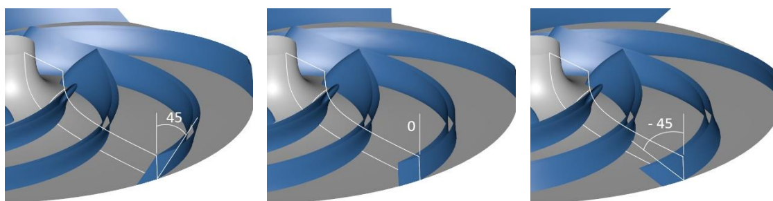
شکل ۵. طراحی پره با سه زاویه لبه خروجی ۰، ۴۵ و -۴۵ درجه نسبت به راستای نصف النهاری.
