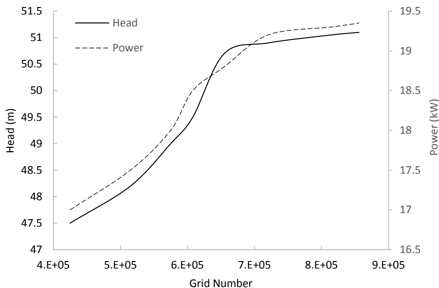
شکل ۷. استقلال نتایج هد و توان از شبکه بندی.
