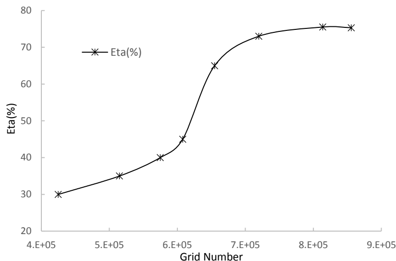
شکل ۸. استقلال نتایج مربوط به راندمان از شبکه بندی
