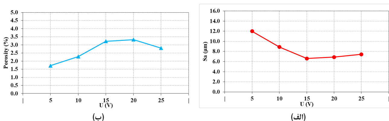
شکل ۷. (الف) تغییرات زبری سطح ( S_a ) و (ب) درصد تخلخل فولاد AISI 304 بر حسب ولتاژ در فرآیند سنگ‌زنی الکتروشیمیایی.
