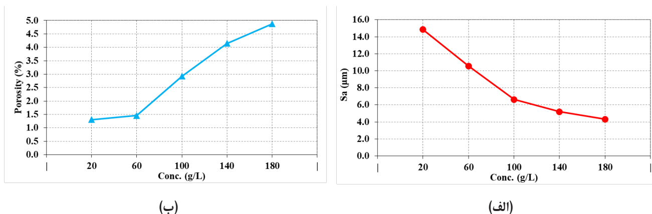
شکل ۶. (الف) تغییرات زبری سطح ( S_a ) و (ب) درصد تخلخل فولاد AISI 304 بر حسب غلظت الکترولیت در فرآیند سنگ‌زنی الکتروشیمیایی.
