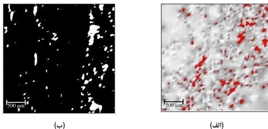
شکل ۵. نمونه‌ای از پردازش تصویر در نرم‌افزار ImageJ برای تعیین درصد تخلخل سطحی: (الف) شناسایی منافذ، (ب) تصویر باینری پس از آستانه‌گذاری و محاسبه مساحت منافذ.
