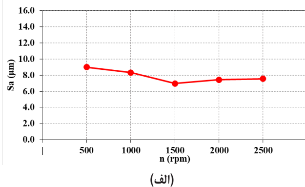
شکل ۸. (الف) تغییرات زبری سطح (Sa) و (ب) درصد تخلخل فولاد AISI 304 بر حسب سرعت چرخش چرخ سنگزنی در فرآیند سنگزنی الکتروشیمیایی.
