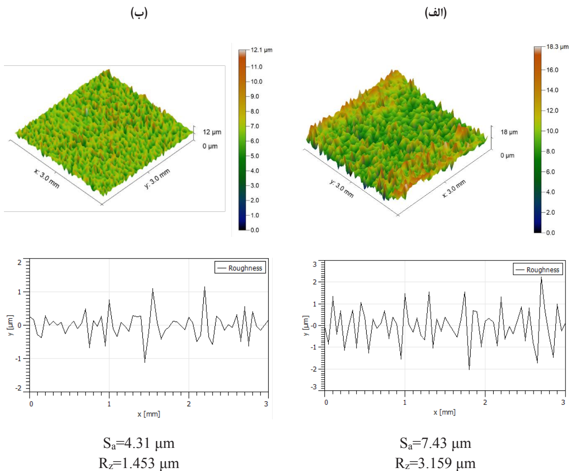
شکل ۴. نمونه‌هایی از نقشه سه‌بعدی سطح فولاد زنگ‌نزن AISI 304 برداشت‌شده توسط پروفایلومتر لیزری.
