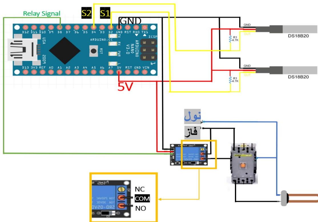
شکل ۳. شماتیک مدار کنترل طراحی شده در نرمافزار فریتزینگ.
