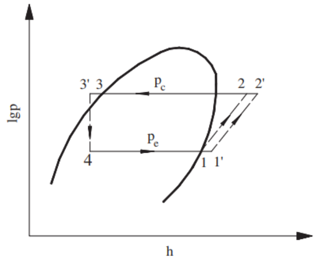
شکل ۲. دیاگرام فشار-انتالپی (P-h) سیکل پمپ حرارتی.
