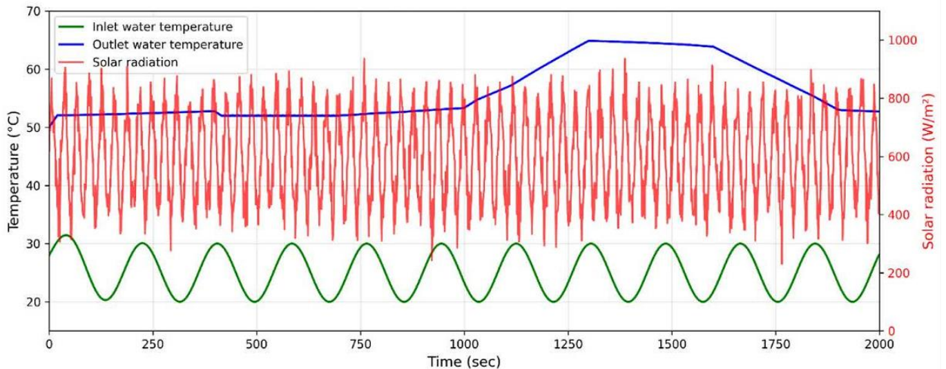
شکل ۱۱. تغییرات دمای آب ورودی، خروجی و تشعشع خورشیدی در برابر زمان
