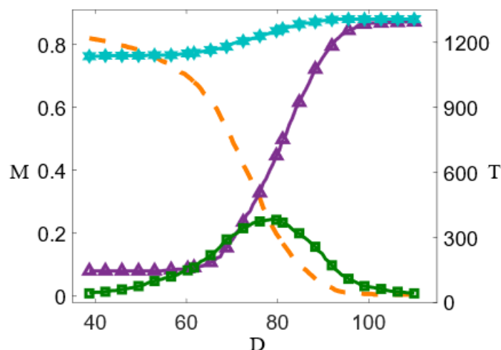
شکل ۱. پروفیل دما (T) و کسر مولی گونه‌ها (M) نسبت به فاصله محوری (D). نمادهای ستاره آبی، مثلث بنفش، مربع سبز و خطچین نارنجی به ترتیب بیانگر دما، \text{CO}_2 ، \text{CO} ، و \text{CH}_4 هستند که بر مبنای داده‌های مرجع [۱۹] بازسازی شده‌اند.
