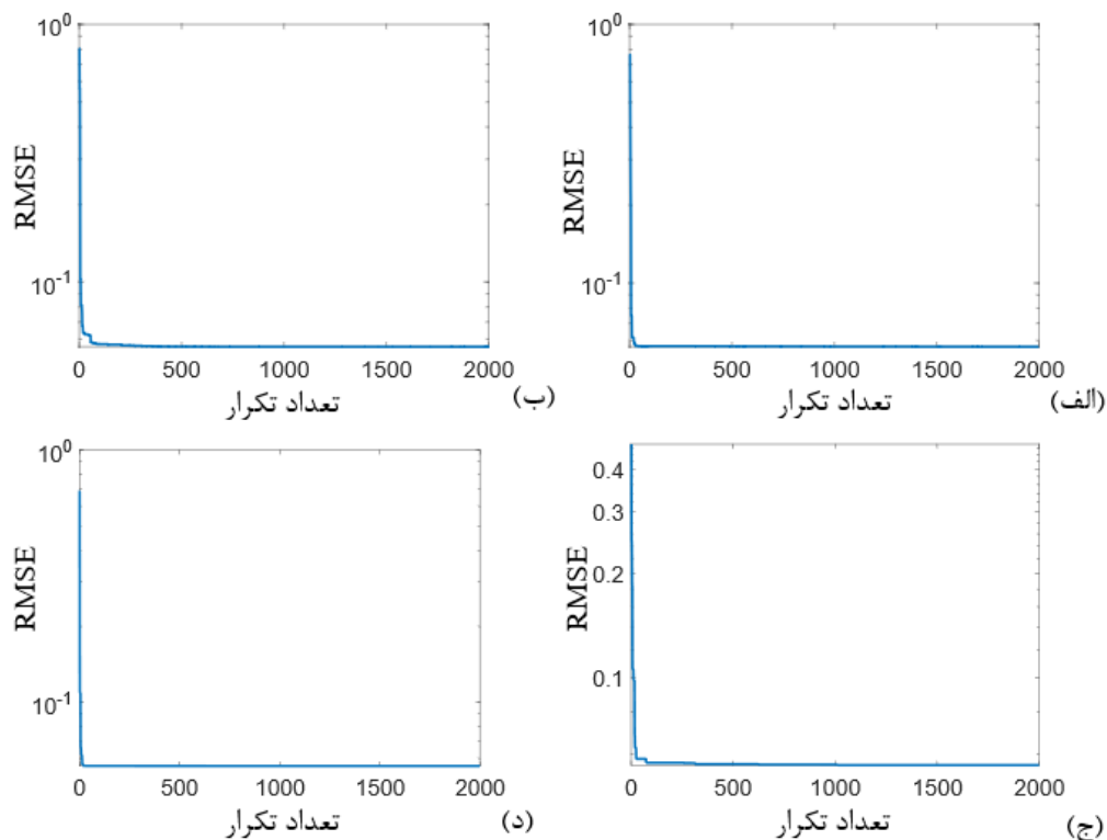
شکل ۳. روند همگرایی الگوریتم‌های نهنگ (الف) ژنتیک، (ب) نهنگ، (ج) گرگ خاکستری و (د) ترکیبی ژنتیک-ازدحام ذرات بر اساس تغییرات ریشه میانگین مربعات خطا بر حسب تعداد تکرار.
