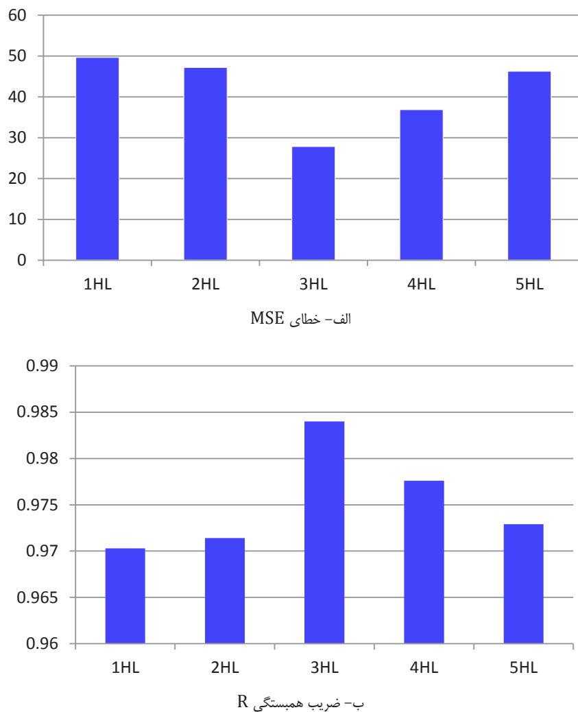
شکل ۹. مقایسه شبکه‌های بهینه در حالات مختلف.
