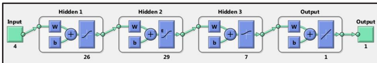
شکل ۱۰. ساختار شبکه MLP بهینه.
