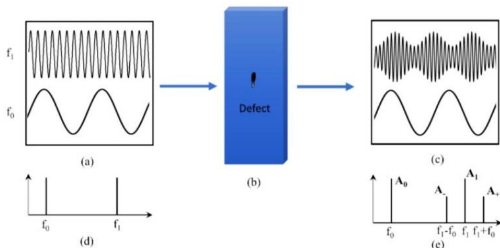
شکل ۲. روش تلفیق ارتعاشی-صوتی: (الف) سیگنال‌های f_1 فرکانس بالا و f_0 فرکانس پایین) به نمونه، (ب) نمونه آزمایشی معیوب، (ج) سیگنال‌های خروجی، (د) طیف توان اولیه در حوزه فرکانس، و (ه) طیف توان خروجی [۳۳].
