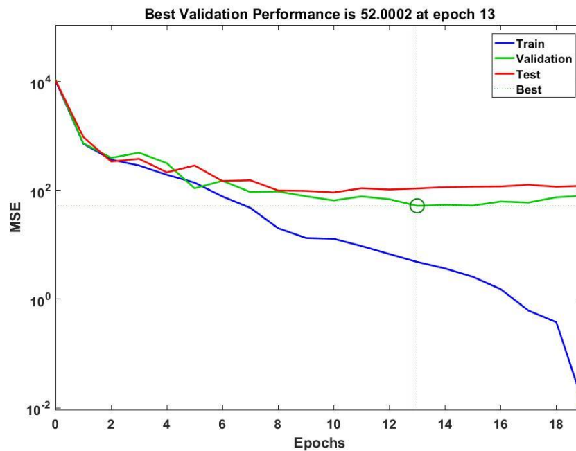
شکل ۱۱. نمودار همگرایی فرایند آموزش شبکه بهینه.
