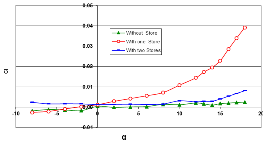
شکل ۲۰: اثرات مخزن سوخت خارجی بر نمودار C_D-\alpha
