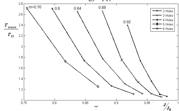
شکل (۳): توزیع تنش برشی در مقاطع چهار سلولی برای a/R = 0.12 (الف) و تنش برشی ماکزیمم برای مقاطع مختلف دایره‌ای (ب)
