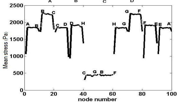
شکل (۱۰): توزیع تنش متوسط در جداره مقطع مستطیلی با سه
