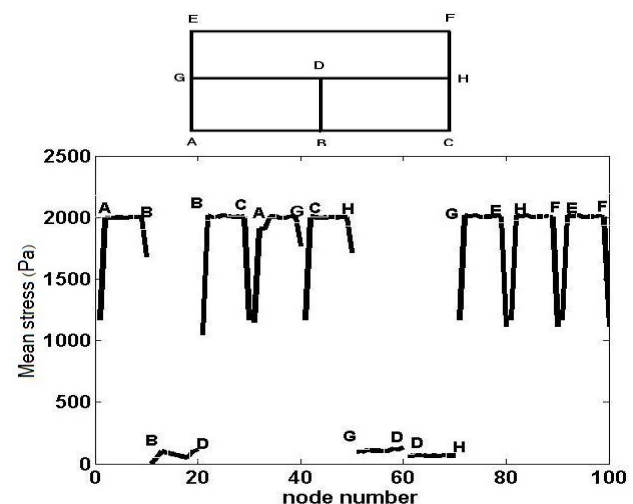
شکل (۱۲): توزیع تنش متوسط در جداره مقطع مستطیلی با سه سلول متفاوت
