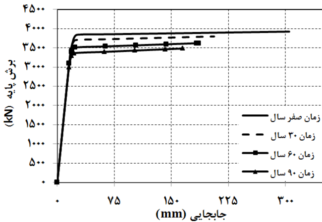
شکل ۱۵: منحنی ظرفیت (بارافزون) عرضی پل
