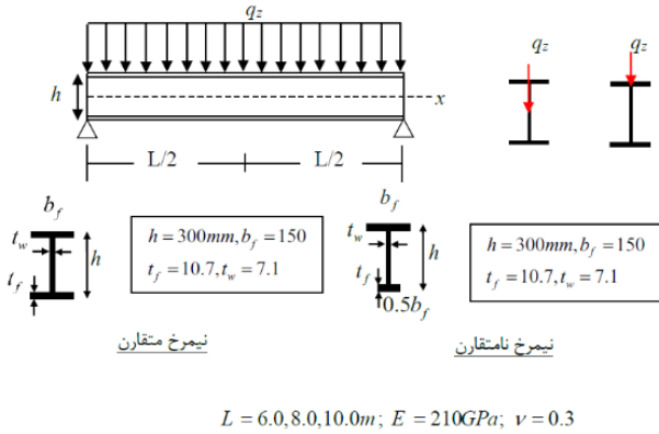
شکل ۶: تیر دو سر مفصل تحت بار گسترده جانبی یکنواخت
