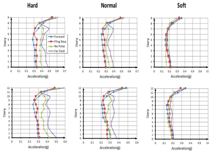
شکل ۹: حداکثر شتاب کف‌های سازه‌های جداسازی شده برای گروه‌های مختلف
