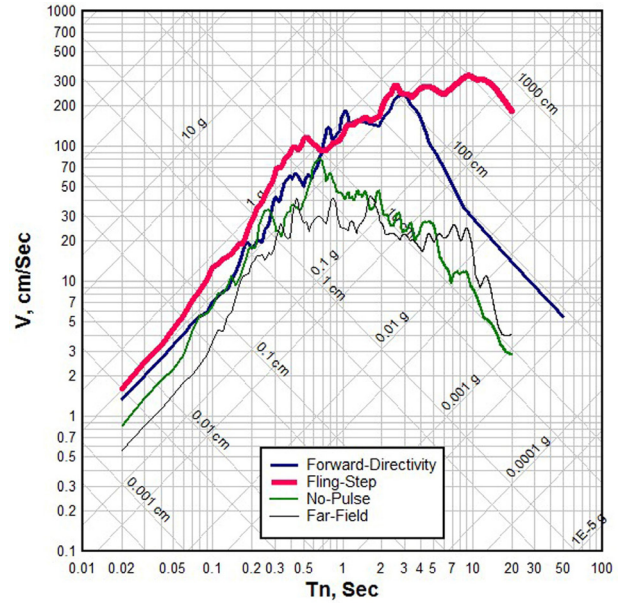
شکل ۵: نمودار سه جانبه (ترکیبی A-V-D) چهار رکورد منتخب از هر دسته رکورد مورد بررسی در این مطالعه به ازای میرایی ۵٪
