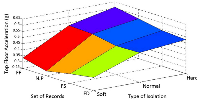
شکل ۱۰: میانگین حداکثر شتاب مطلق بام تحت اثر چهار دسته رکورد در مقابل تغییرات سختی جداساز برای سازه ۹ طبقه
